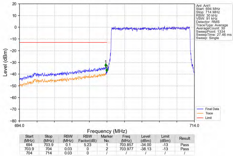
Band17_10MHz_QPSK_LCH_709MHz_RB_50_0_NTNV
