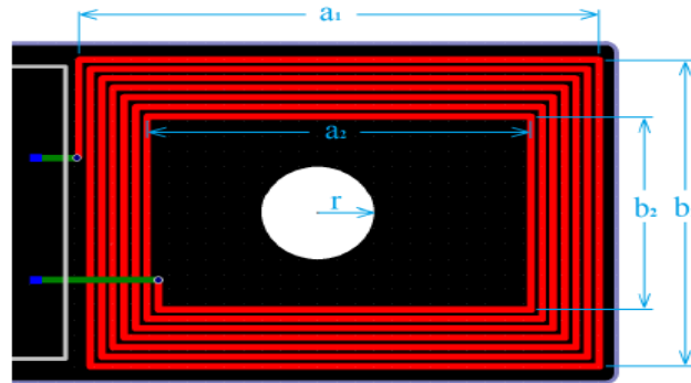
尺寸参数( SIZE PARAMETERS)
