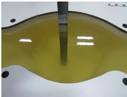
Body(1750MHz)_16.2cm
