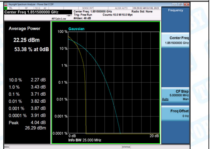
Band2-3MHz-QPSK-18615-1RB#0-PASS
