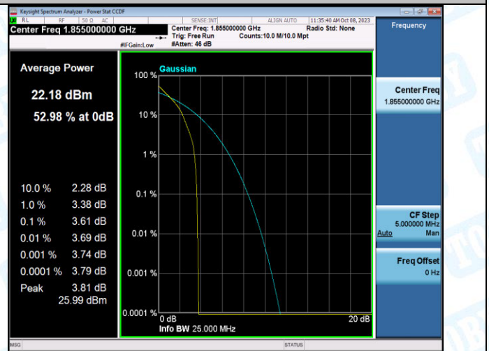
Band2-10MHz-QPSK-18650-1RB#0-PASS
