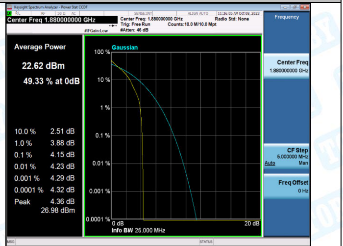
Band2-10MHz-QPSK-18900-1RB#0-PASS
