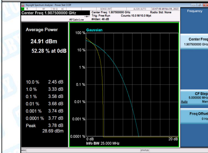
Band2-5MHz-QPSK-19175-1RB#0-PASS
