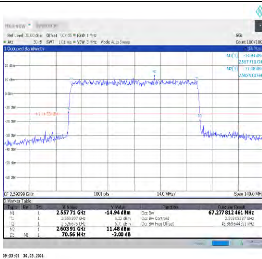
1-N41-30-70-M-9-CP-256QAM-Outer_Full-189@0-A nt1-67.278-70.560-≤70-PASS
