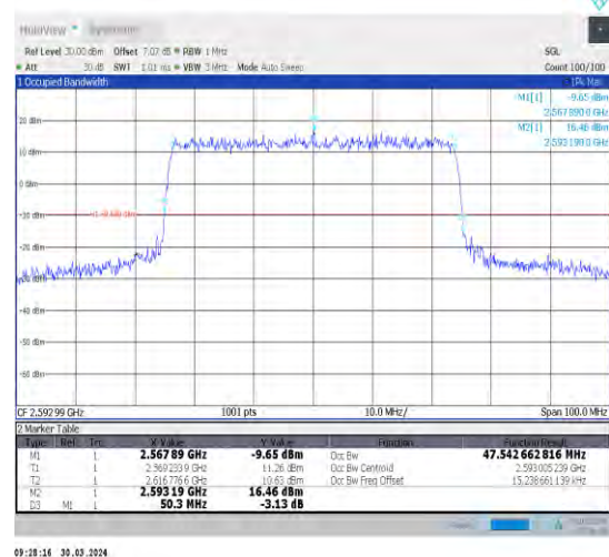
1-N41-30-50-M-6-CP-QPSK-Outer_Full-133@0-A nt1-47.543-50.300-≤50-PASS
