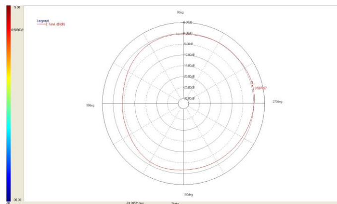
YZ-Plane 2442MHz
