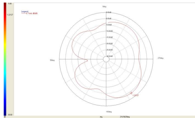
XY-Plane 2442MHz
