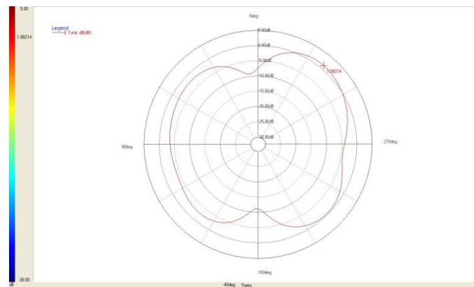
XZ-Plane 2442MHz
