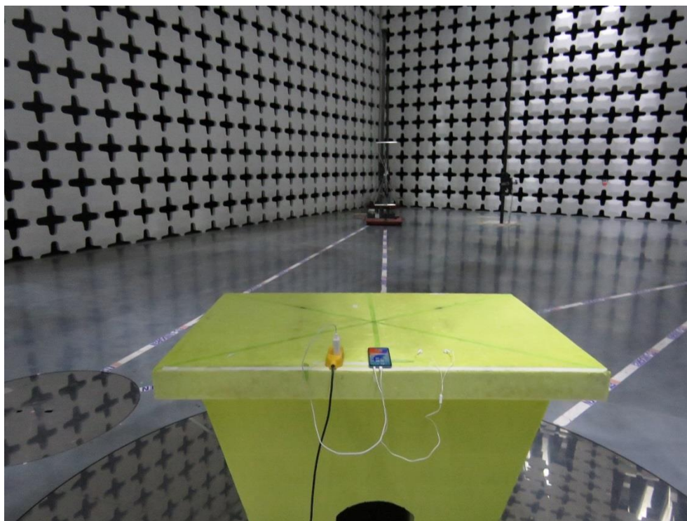
Part15B_RE_L1
