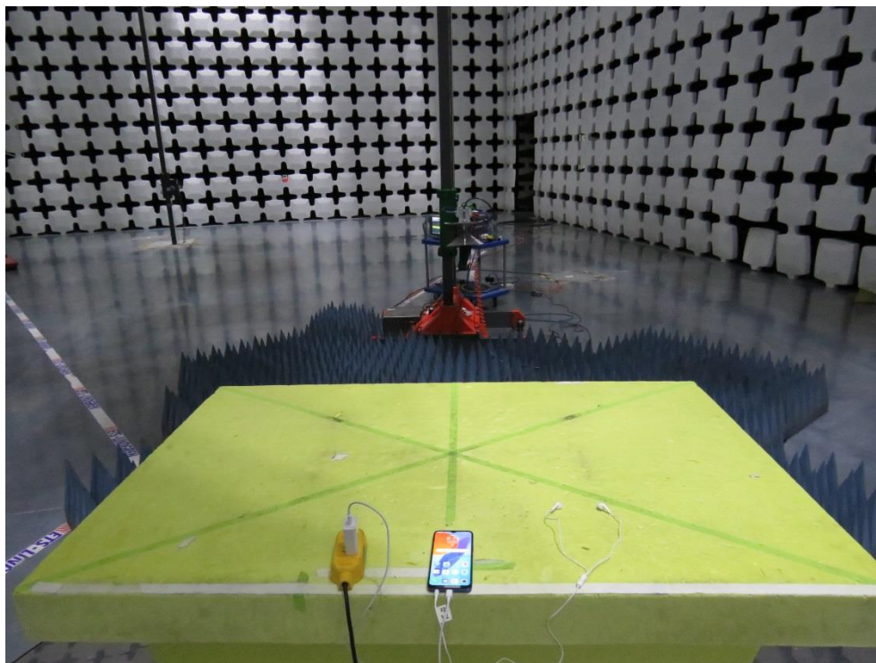
Part15B_RE_H1
