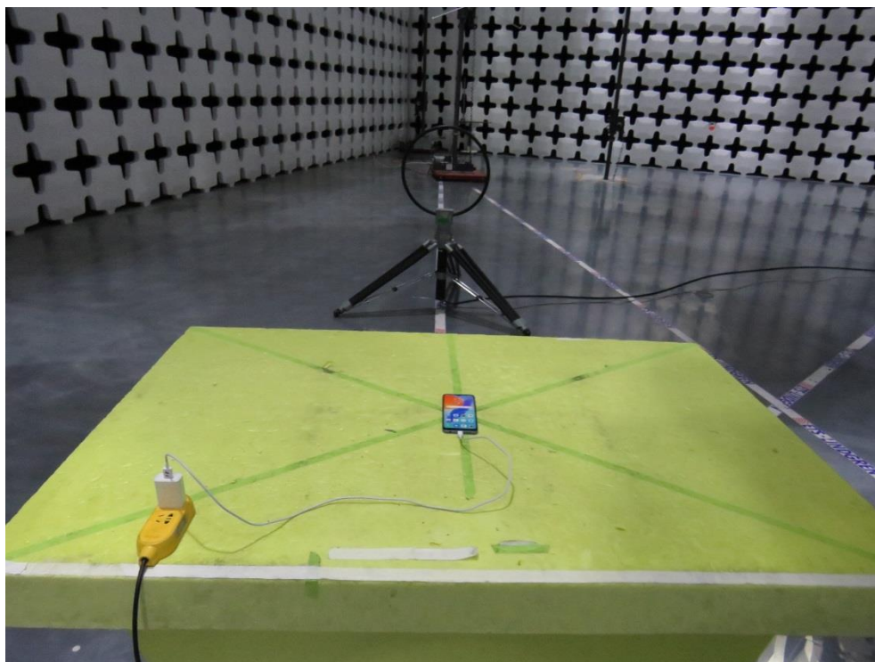
Part15C_15E_RE_L2
