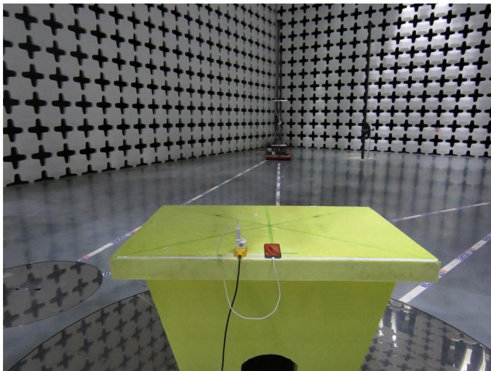
Part15C_15E_RE_L
