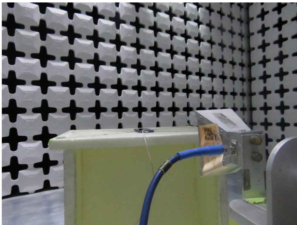
Part15C_15E_RE_H
