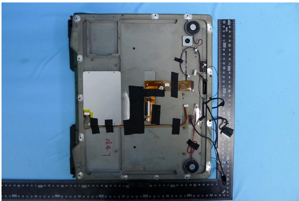
(65) EUT Photo
