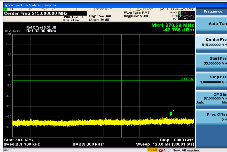
Band4-10MHz-QPSK-20000-1RB#0-30~1000MHz
