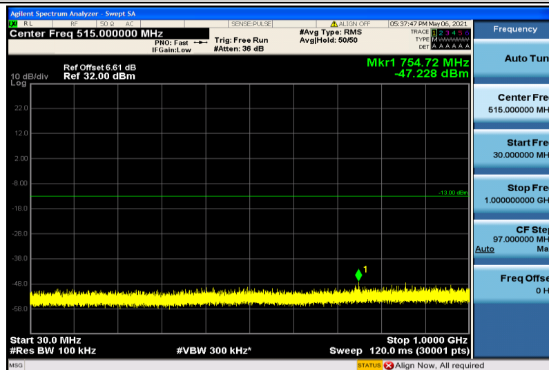
Band2-20MHz-QPSK-18900-1RB#0-30~1000MHz
