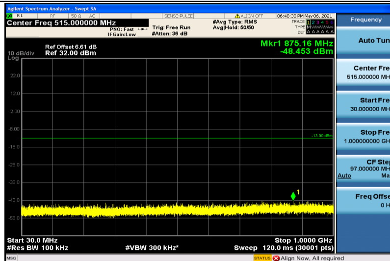
Band4-3MHz-QPSK-19965-1RB#0-30~1000MHz
