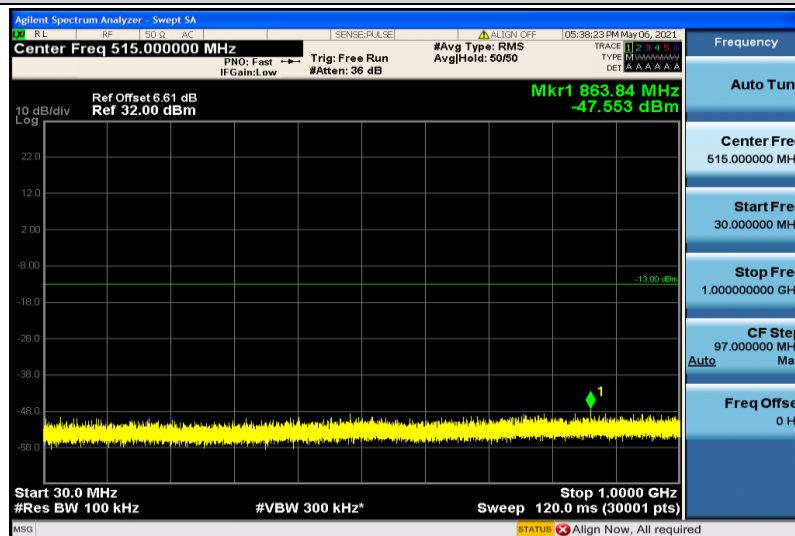
Band2-20MHz-16QAM-18900-1RB#0-30~1000MHz
