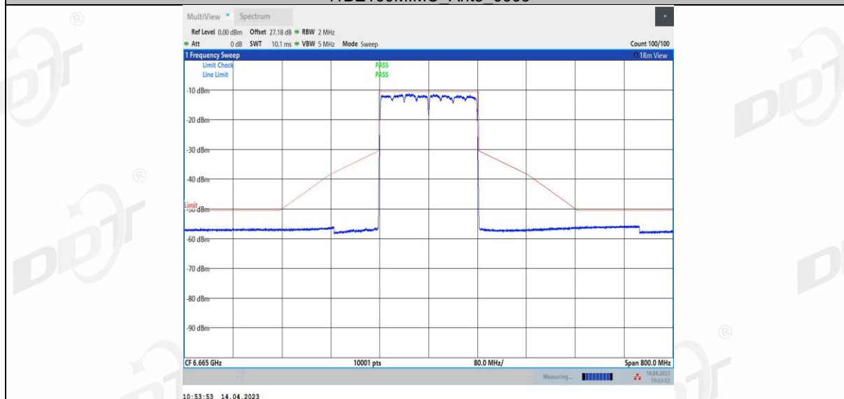
11BE160MIMO Ant4 6665
