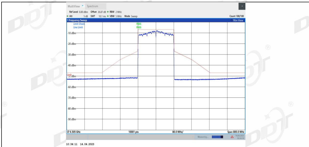
11BE160MIMO Ant4 6505
