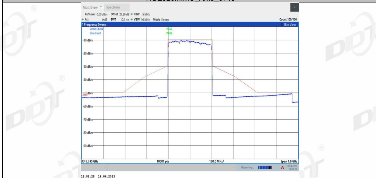
11BE320MIMO Ant4 6745
