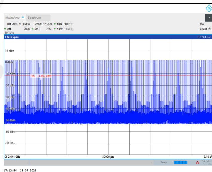
3DH3_Ant1_Hop
