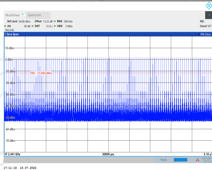
3DH1_Ant1_Hop
