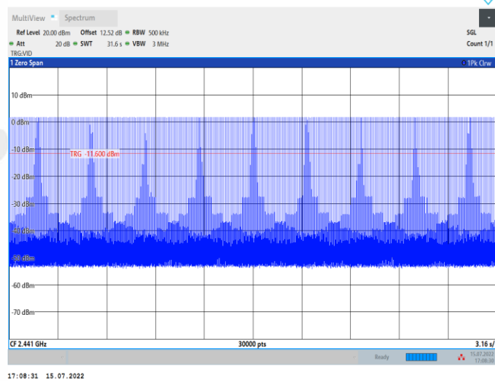
2DH3_Ant1_Hop
