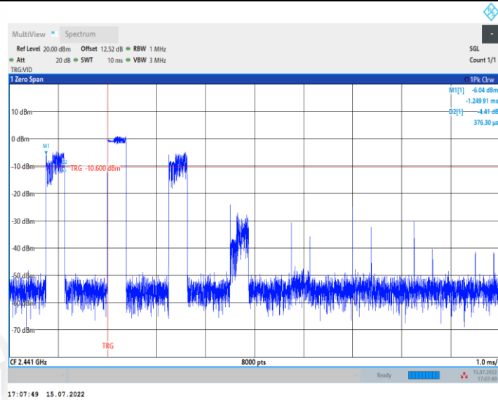
2DH1_Ant1_Hop
