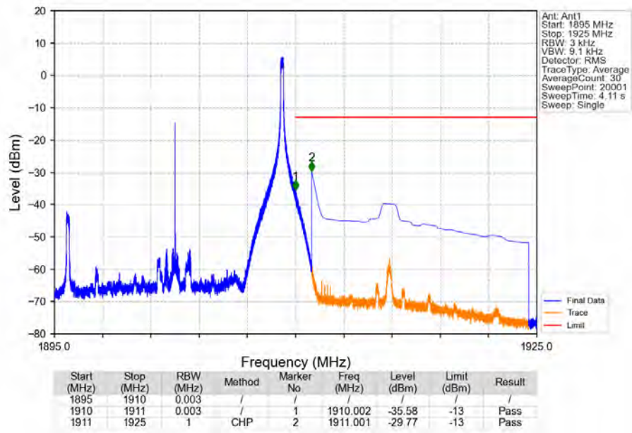
Band2_15MHz_QPSK_HCH_1902.5MHz_RB_1_74_NTNV
