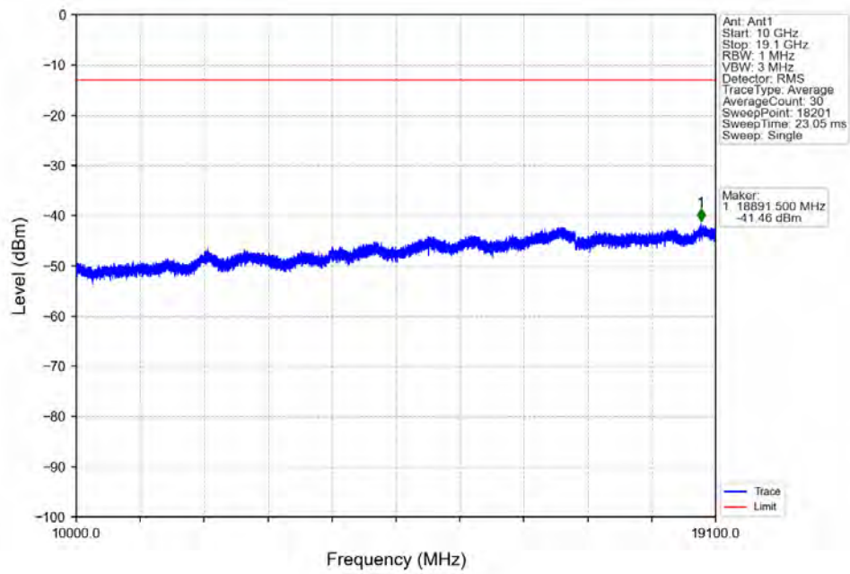
Band2_15MHz_QPSK_HCH_1902.5MHz_RB_1_74_NTNV
