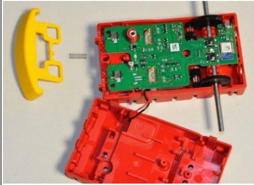
EUT OPEN
