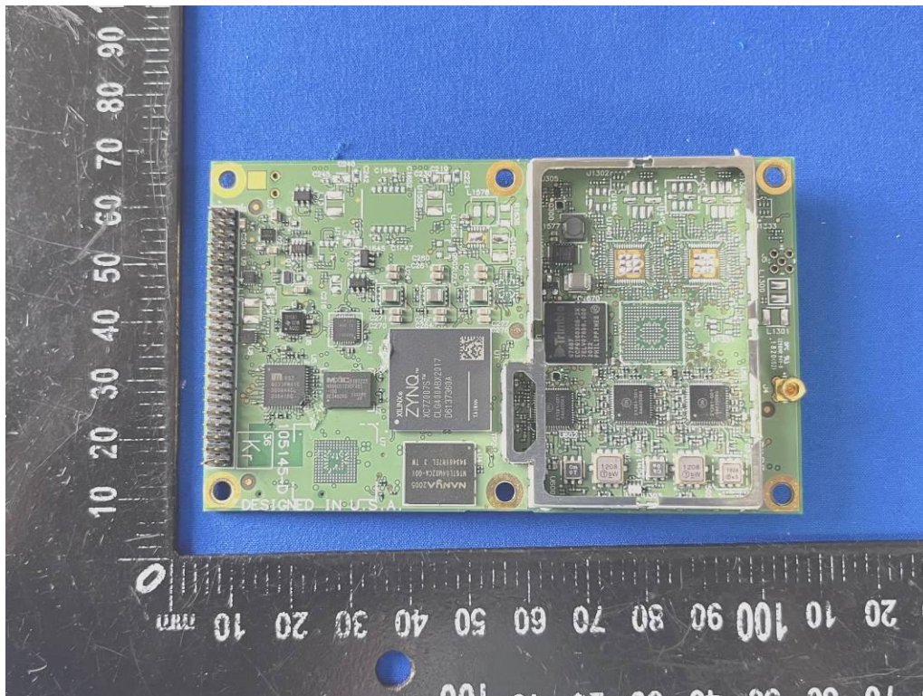
Internal view(PA-3 Pro)
