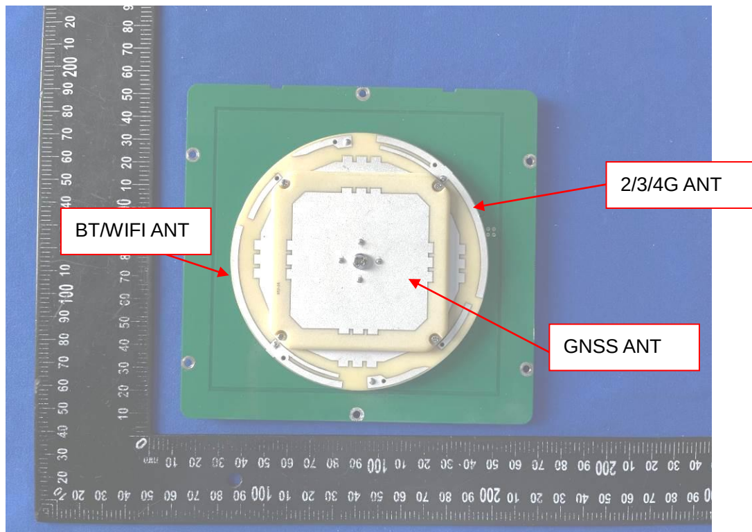
Internal view(PA-3 Pro)
