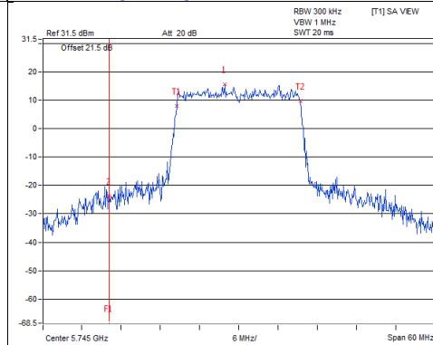
802.11ax (HE20) / Chain 3 : CH149
