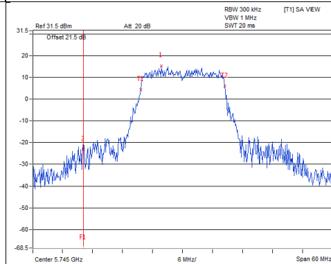
802.11ax (HE20) / Chain 1 : CH149
