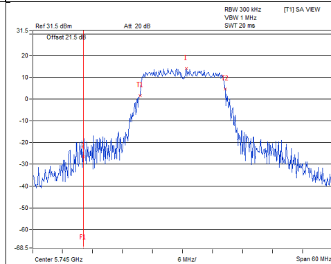
802.11a / Chain 3 : CH149
