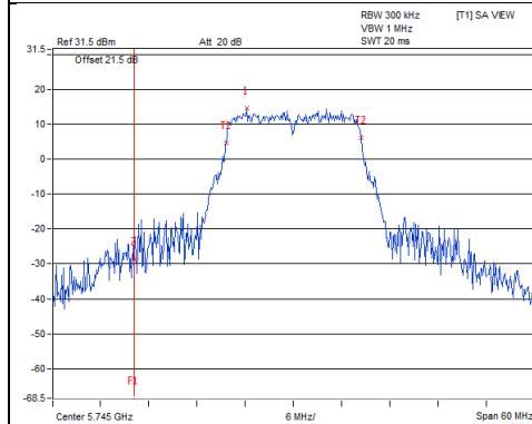
802.11a / Chain 2 : CH149
