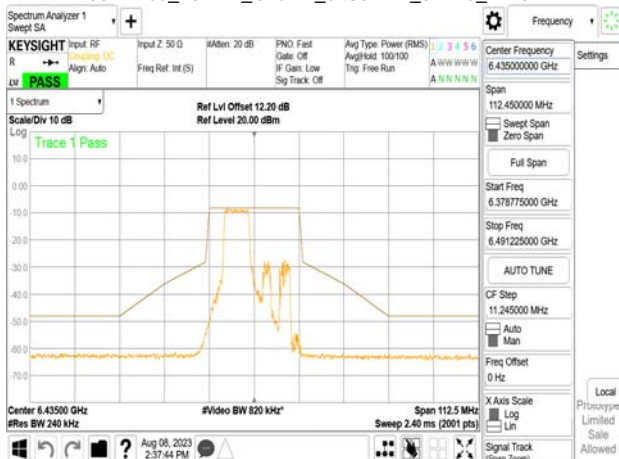
802.11be_20MHz_Chain1_6435MHz_52+26_MRUI
