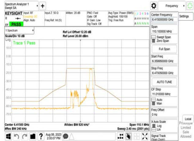
802.11be_20MHz_Chain1_6415MHz_RU52_40
