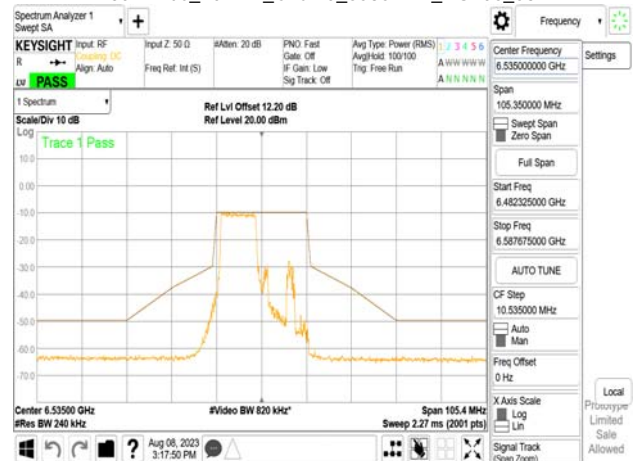
802.11be_20MHz_Chain0_6535MHz_RU106_53
