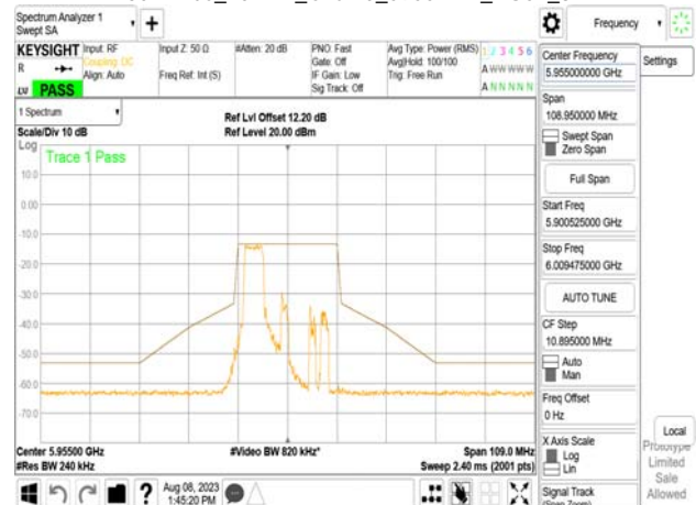
802.11be_20MHz_Chain0_5955MHz_RU52_37
