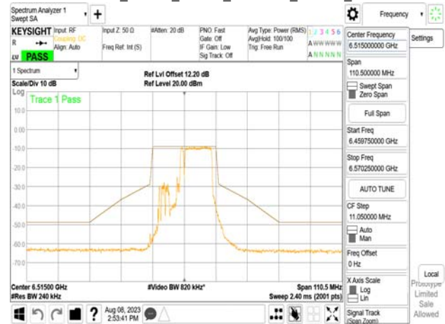
802.11be_20MHz_Chain0_6515MHz_52+26_MRU3
