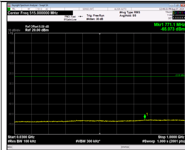
2-2-5MHz-20MHz-QPSK-QPSK-18808-18925-25RB#0-1 00RB#0-30~1000MHz-PASS
