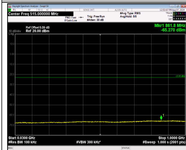
2-2-5MHz-20MHz-QPSK-QPSK-18983-19100-1RB#0-1R B#99-30~1000MHz-PASS
