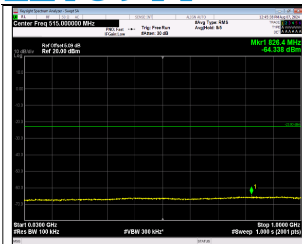
2-2-5MHz-20MHz-QPSK-QPSK-18808-18925-1RB#0-0R B#0-30~1000MHz-PASS
