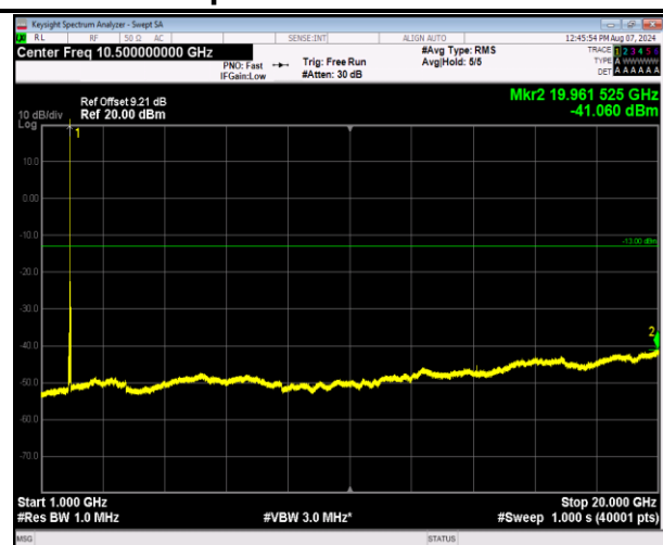
2-2-5MHz-20MHz-QPSK-QPSK-18808-18925-1RB#0-0R B#0-1000~20000MHz-PASS
