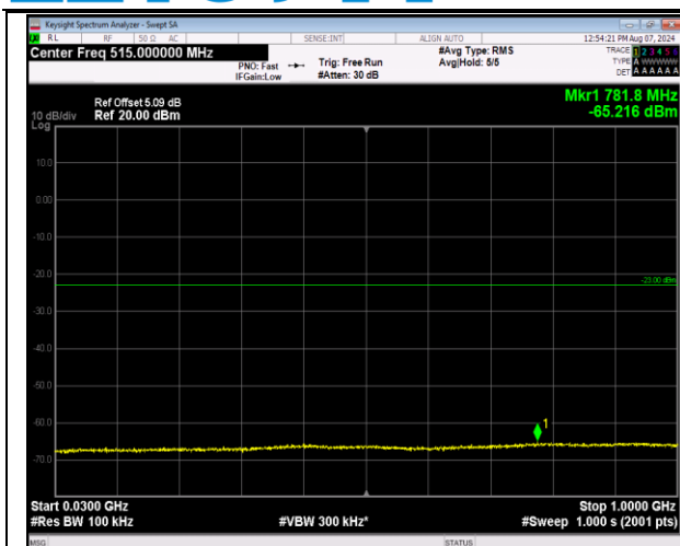
2-2-5MHz-20MHz-QPSK-QPSK-18983-19100-25RB#0-1 00RB#0-30~1000MHz-PASS
