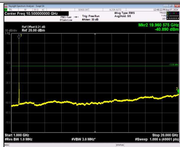
2-2-5MHz-20MHz-QPSK-QPSK-18808-18925-1RB#0-1R B#99-1000~20000MHz-PASS
