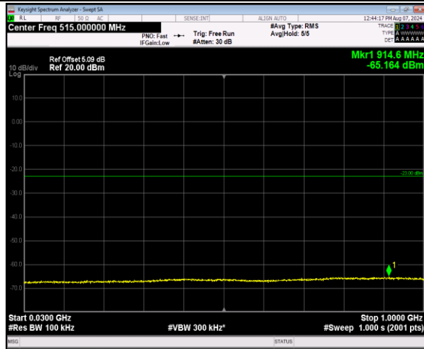
2-2-5MHz-20MHz-QPSK-QPSK-18633-18750-25RB#0-1 00RB#0-30~1000MHz-PASS
