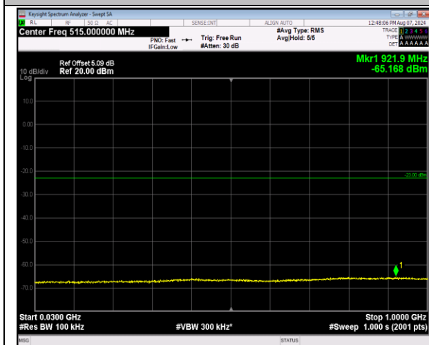
2-2-5MHz-20MHz-QPSK-QPSK-18808-18925-1RB#0-1R B#99-30~1000MHz-PASS
