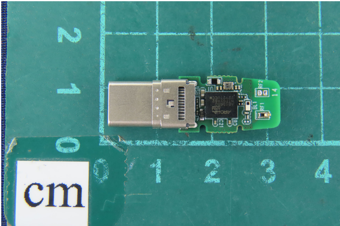
(4) EUT Photo
