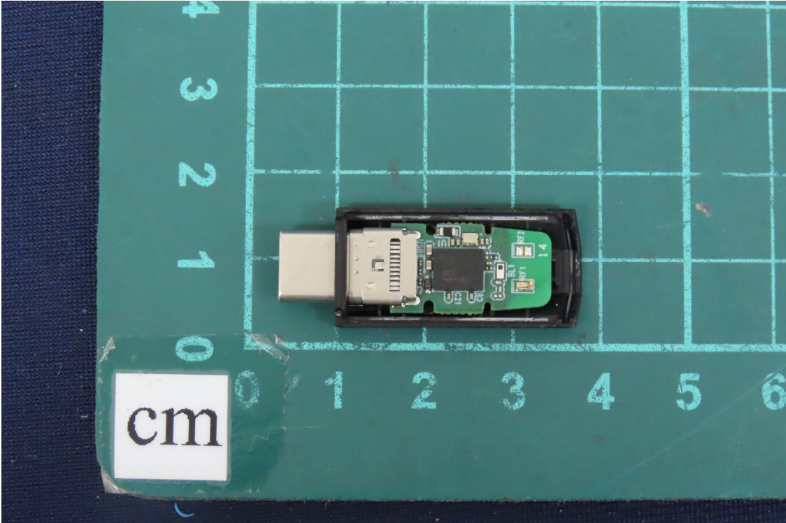
(2) EUT Photo
