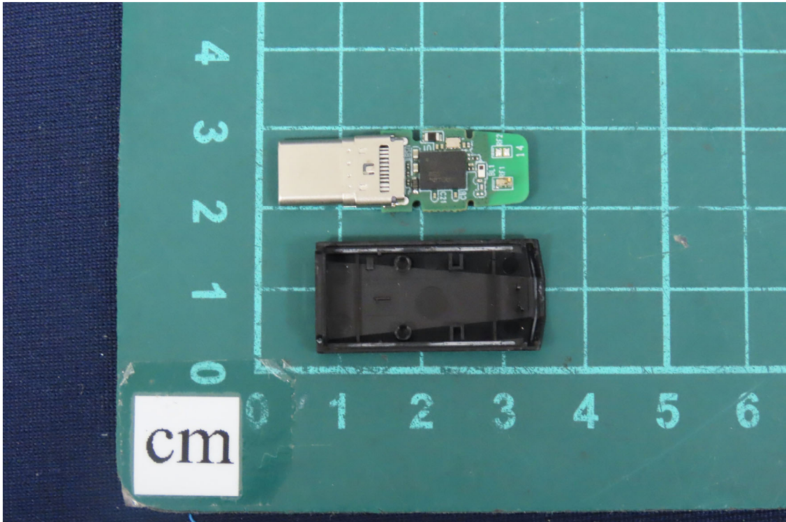
(3) EUT Photo
