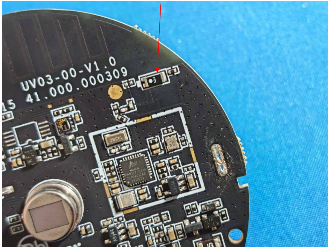
Lora Antenna
