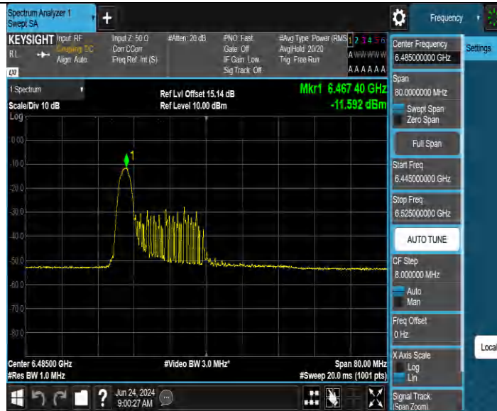
11BE40MIMO_Ant2_6485_26Tone_RU0
