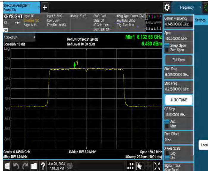
11BE80MIMO_Ant2 6145
