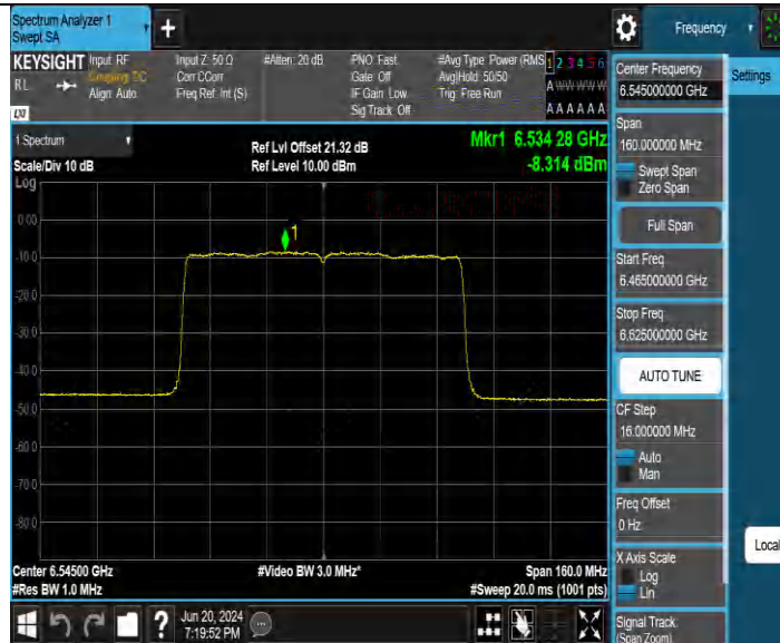
11BE80MIMO_Ant2 6545
