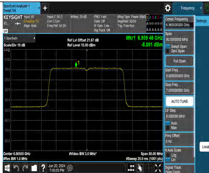
11BE40MIMO_Ant2_6965
