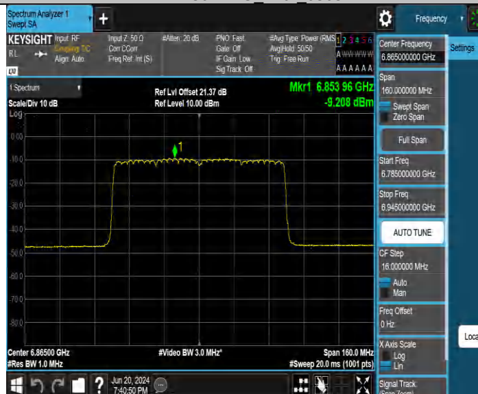
11BE80MIMO_Ant2_6865
