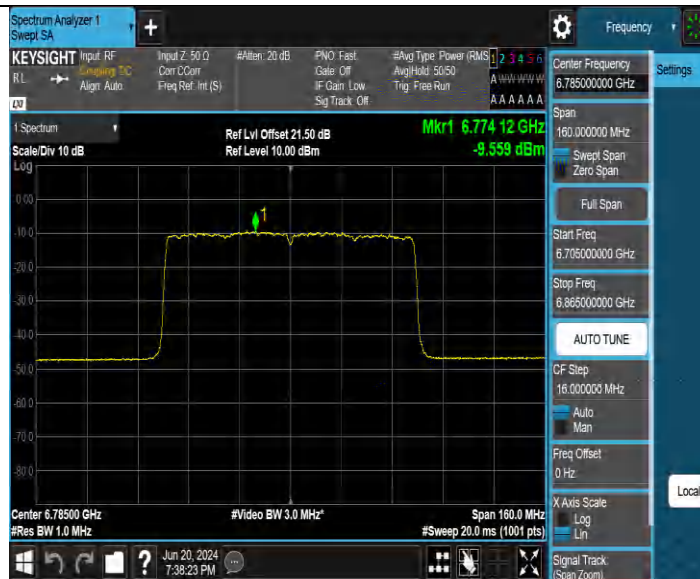
11BE80MIMO_Ant2_6785
