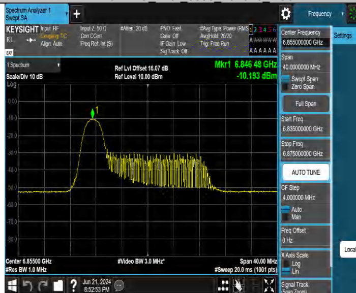
11BE20MIMO_Ant3_6855_26Tone_RU0
