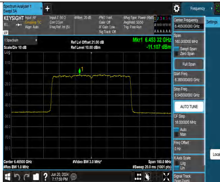
11BE80MIMO_Ant3_6465
