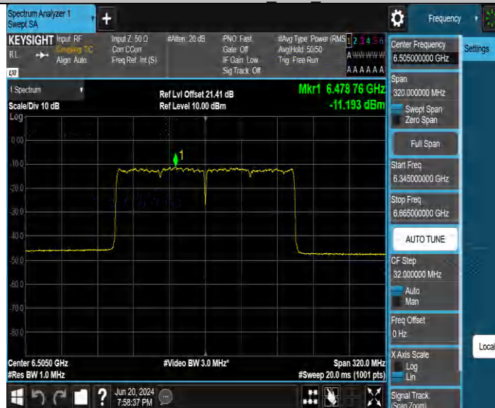
11BE160MIMO Ant3 6505
