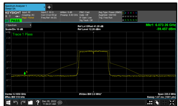
Figure 87 - A(Core 0) 802.11ax HE40 SU 6165 MHz (CH43)
