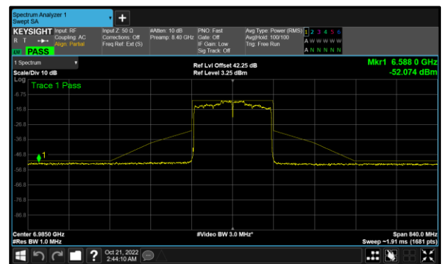
Figure 89 - B(Core 1) 802.11ax HE160 SU 6985 MHz (CH207)
