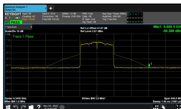
<ImageCaption> - A(Core 0) 802.11ax HE160 SU 6345 MHz (CH79)
