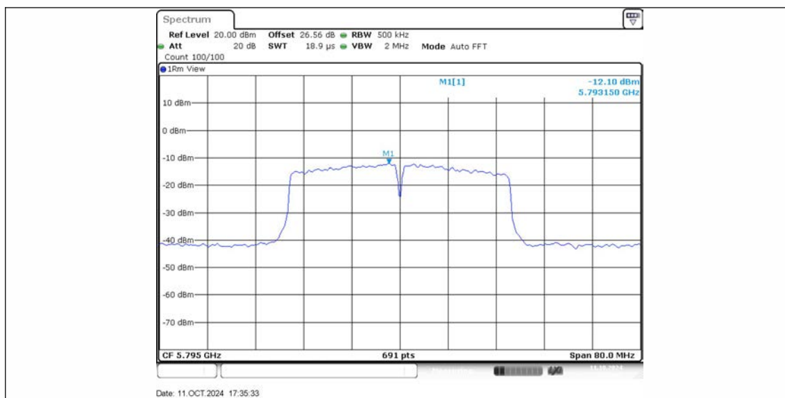
11AC40MIMO_Ant2_5795
