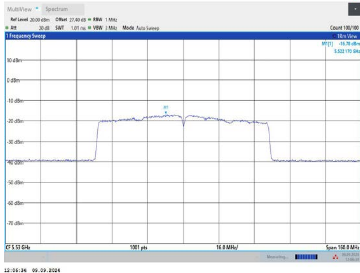
11AC80MIMO_Ant2_5530
