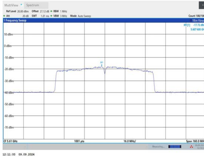
11AC80MIMO_Ant2_5610
