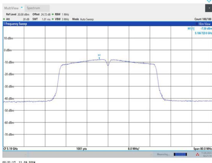
11N40MIMO_Ant2_5190
