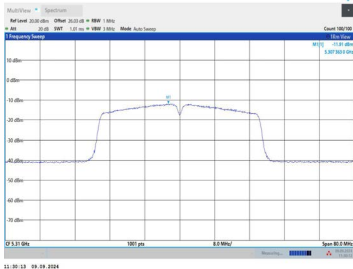
11AC40MIMO_Ant2_5310
