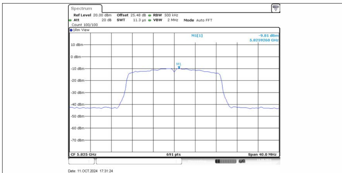
11AC20MIMO_Ant2_5825
