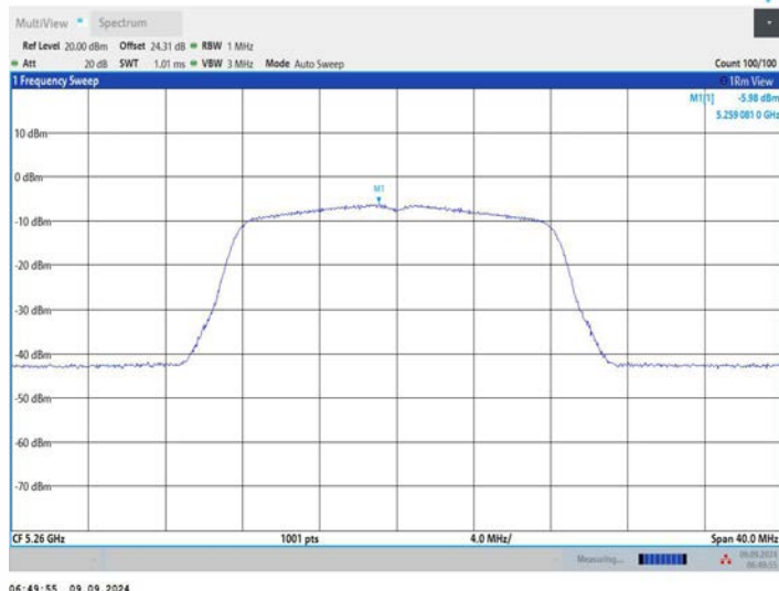
11A_Ant2_5260
