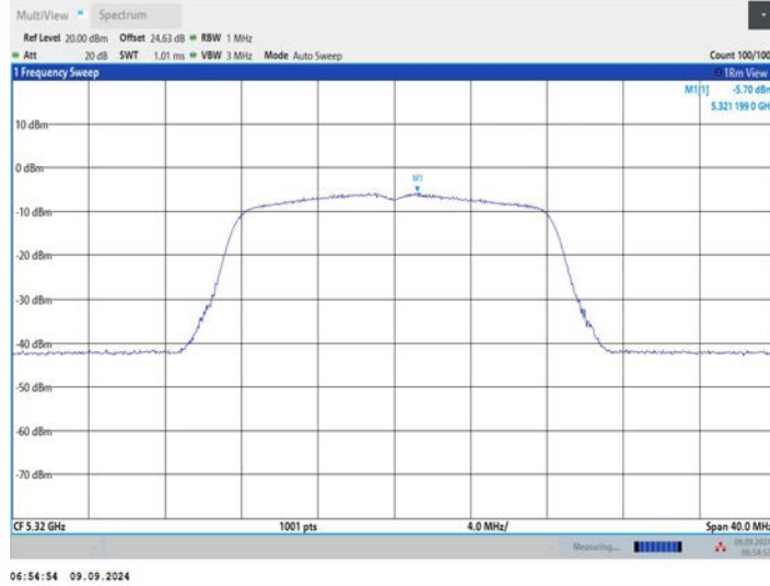
11A_Ant2_5320
