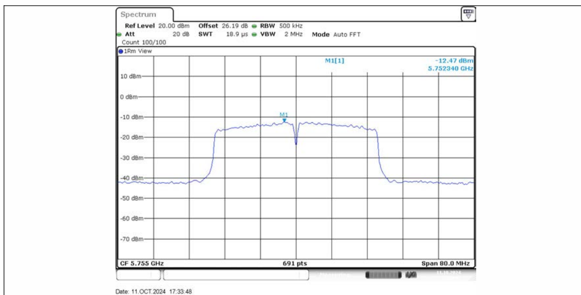
11AC40MIMO_Ant2_5755
