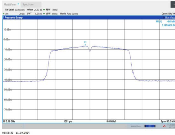
11AC40MIMO_Ant2_5190
