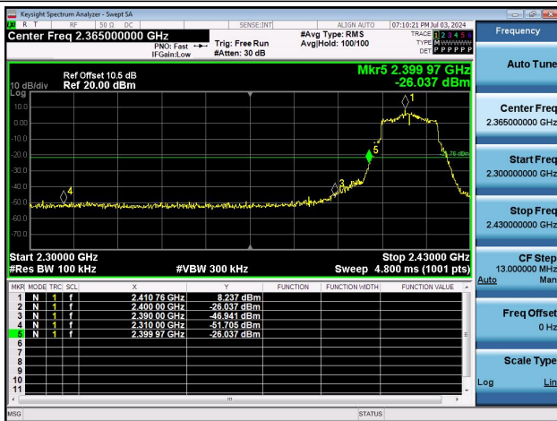
11G-Ant0-2412-PASS
