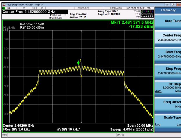
11N20MIMO-Ant0-2462-PASS
