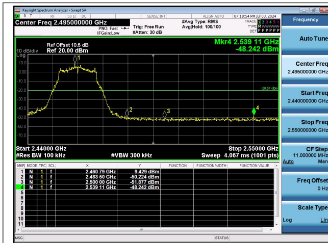
11G-Ant0-2462-PASS
