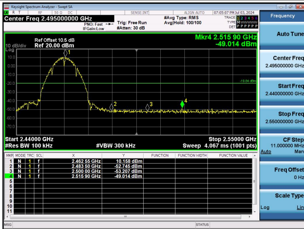
11B-Ant0-2462-PASS
