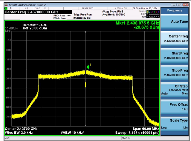
11AX40MIMO-Ant1-2437-PASS
