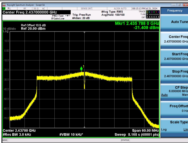
11AX40MIMO-Ant0-2437-PASS
