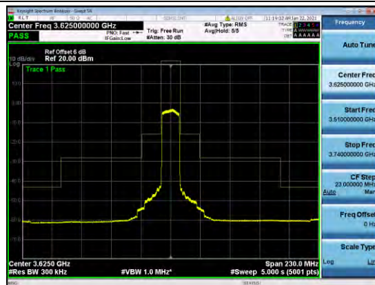
B48-15M-MASK-M-Q64
