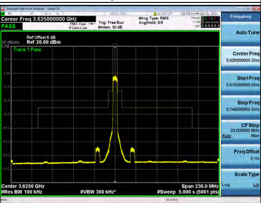
B48-5M-MASK-H-Q16
