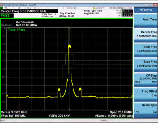
B48-5M-MASK-M-QPSK
