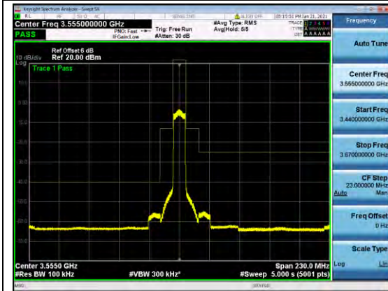
B48-10M-MASK-M-QPSK
