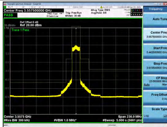
B48-15M-MASK-M-QPSK
