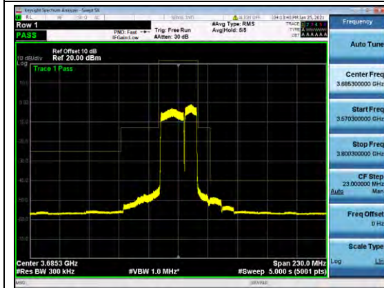
B48-20-15-MASK-L-Q16
