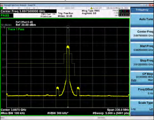
B48-10M-MASK-L-QPSK
