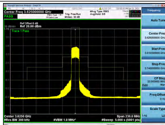
B48-15M-MASK-H-Q16
