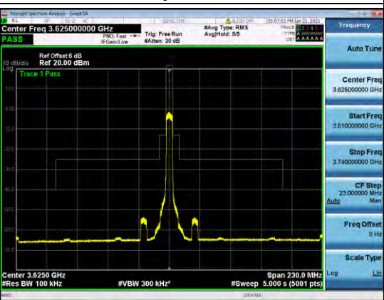
B48-5M-MASK-M-Q64
