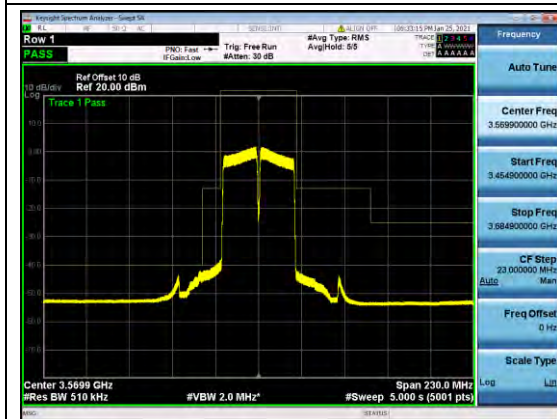
B48-20-20-MASK-M-Q16
