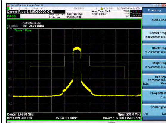
B48-15M-MASK-H-QPSK
