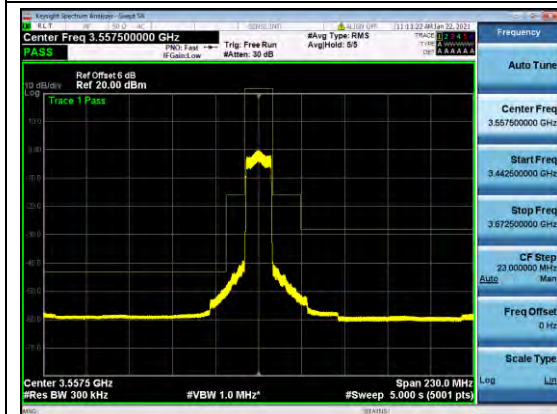
B48-15M-MASK-M-Q16
