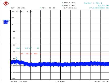
B48-20M-CSE-H-Q64-3
