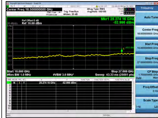
B48-20M-CSE-H-Q64-2
