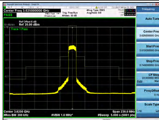
B48-15M-MASK-H-Q16
