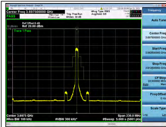
B48-10M-MASK-L-Q16
