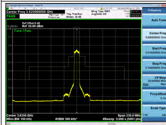
B48-10M-MASK-H-Q16
