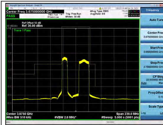
B48-NON-15-20-MASK-L-Q16
