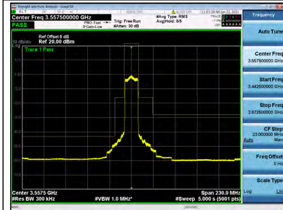
B48-15M-MASK-L-Q64
