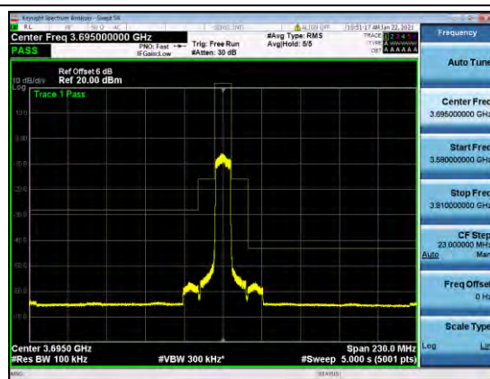
B48-15M-MASK-L-Q16
