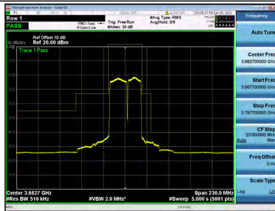
B48-20-20-MASK-L-Q16
