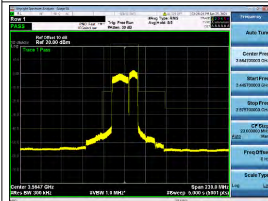
B48-20-10-MASK-M-Q16
