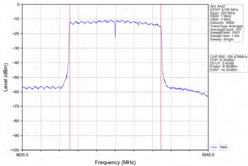
802.11ax(HEW160) MCH_6185MHz_2xRU996_Left_Ant2_NTNV
