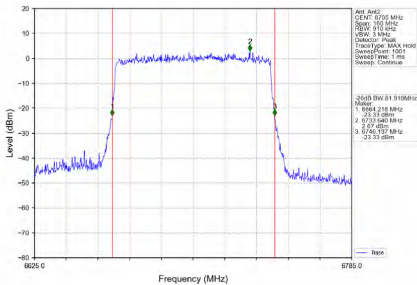
802.11ax(HEW80)_MCH_6705MHz_RU996_Left_Ant2_NTNV
