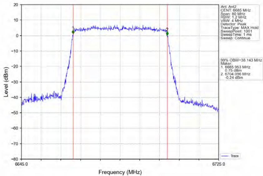
802.11ax(HEW40)_MCH_6685MHz_RU484_Left_Ant2_NTNV
