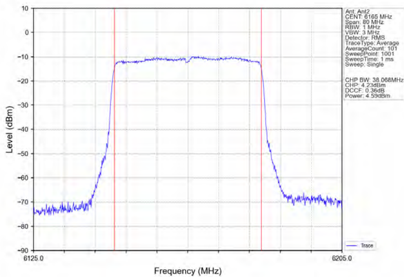
802.11ax(HEW40)_MCH_6165MHz_RU484_Left_Ant2_NTNV
