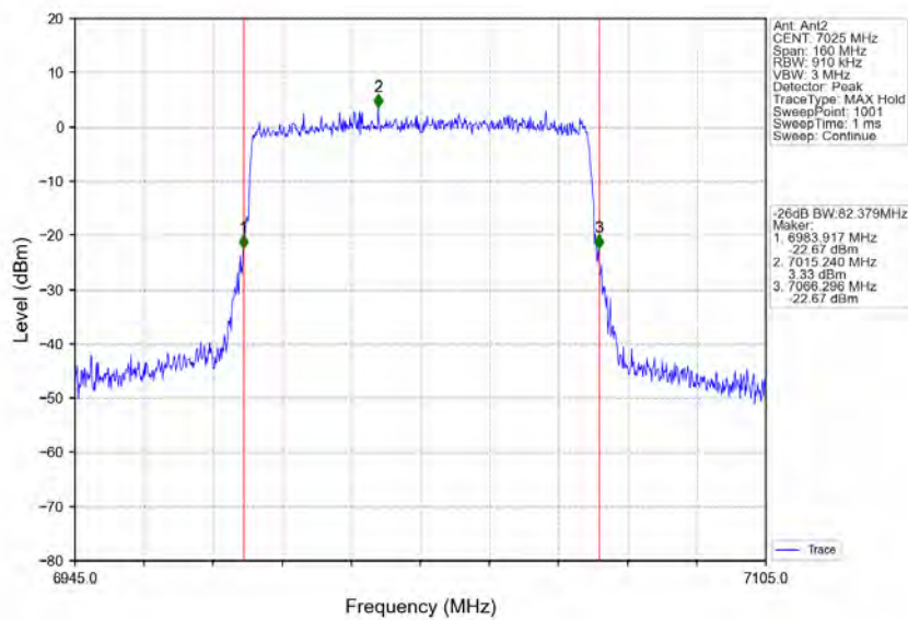
802.11ax(HEW80) HCH 7025MHz RU996 Left Ant2 NTVN
