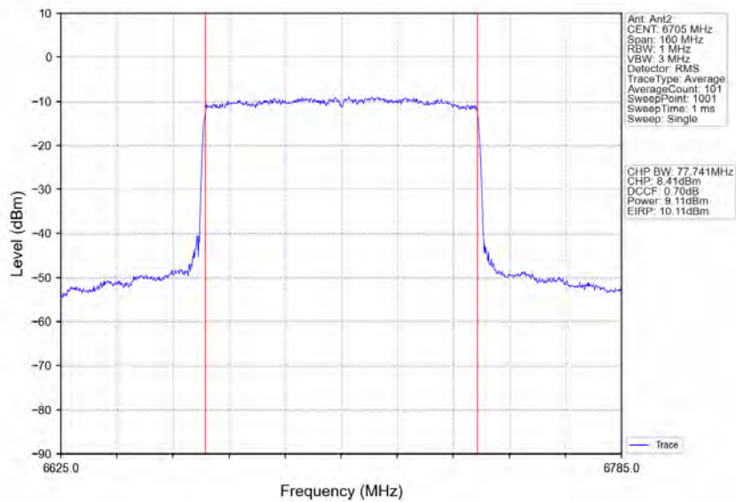
802.11ax(HEW80) MCH 6705MHz RU996 Left Ant2 NTVN
