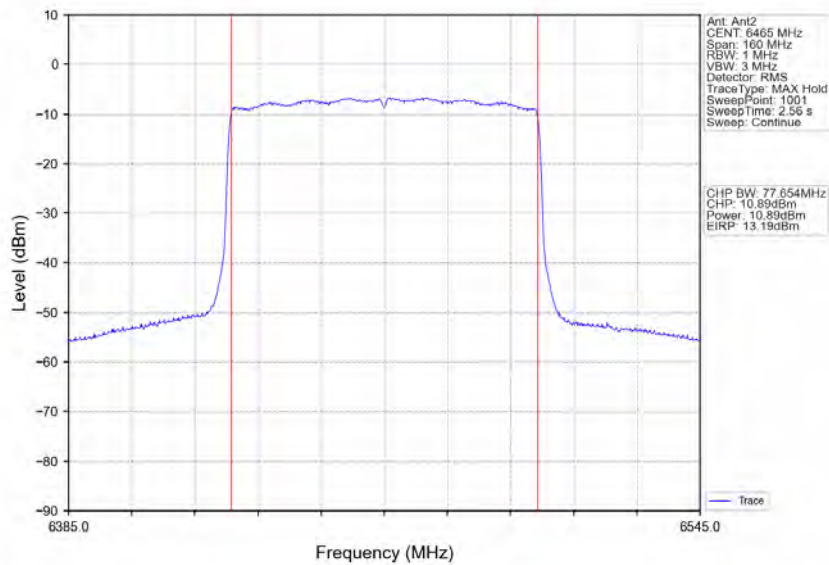
802.11ax(HEW80)_LCH_6465MHz_RU996_Left_Ant2_NTNV
