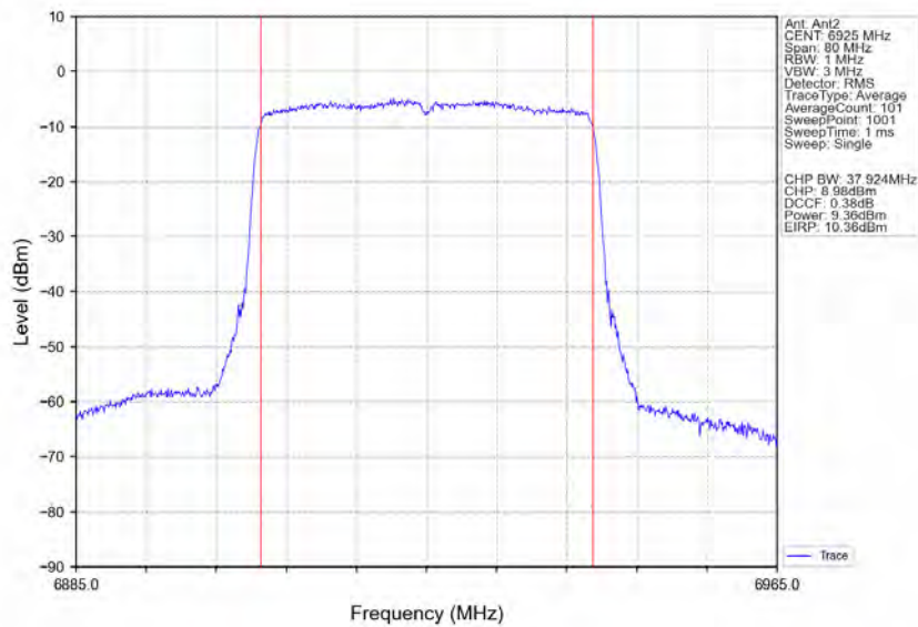
802.11ax(HEW40)_LCH_6925MHz_RU484_Left_Ant2_NTNV
