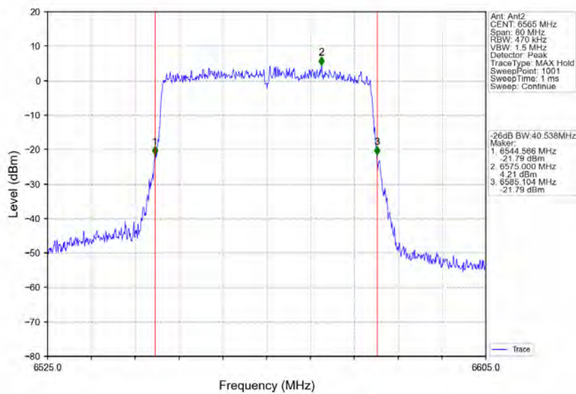
802.11ax(HEW40)_LCH_6565MHz_RU484_Left_Ant2_NTNV
