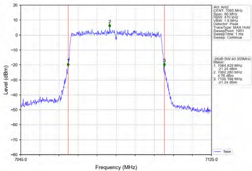
802.11ax(HEW40) HCH 7085MHz RU484 Left Ant2 NTVN
