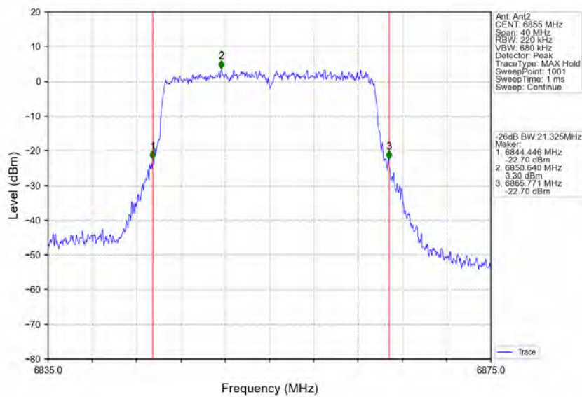
802.11ax(HEW20) HCH 6855MHz RU242 Left Ant2 NTVN
