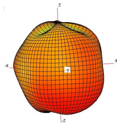
1800MHz
