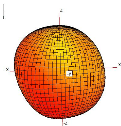
800MHz
