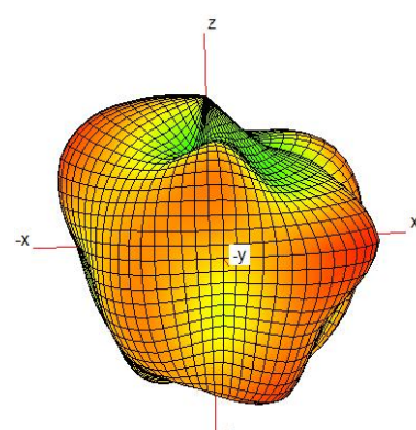
2100MHz
