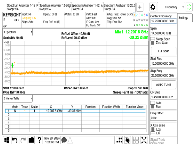
BLE_2M_2480MHz
