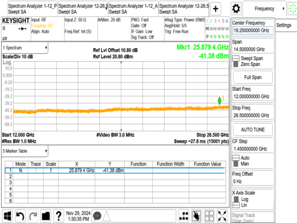
BLE_1M_2442MHz
