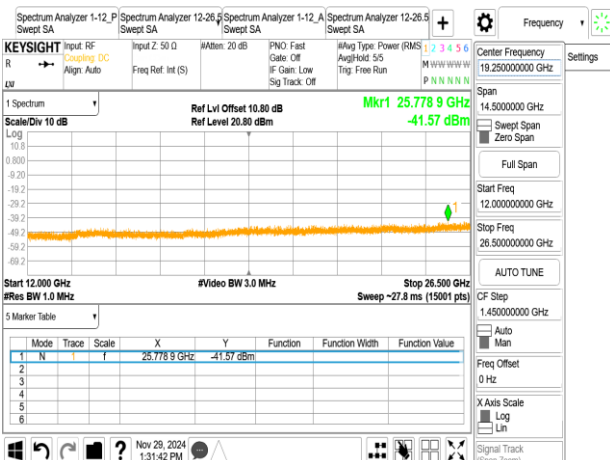
BLE_1M_2480MHz
