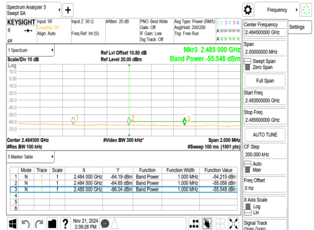
CBE_BLE_500K_2480MHz
