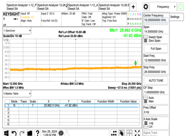
BLE_2M_2480MHz
