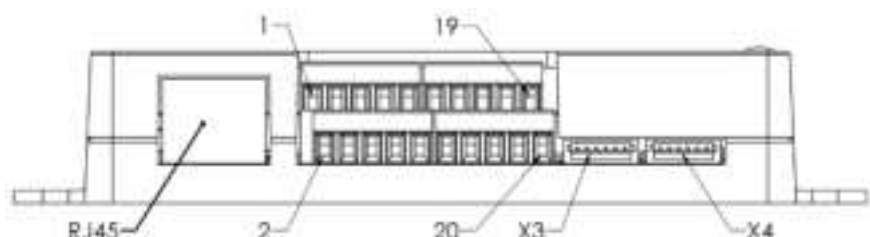
Apexx e-Box
