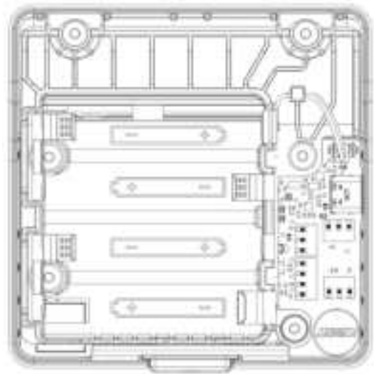
Faceplate (Interior)
