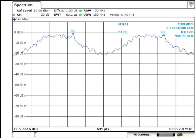
GFSK
