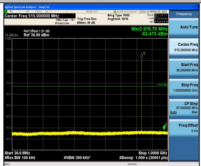
EGPRS850-190-8-30~1000MHz-PASS
