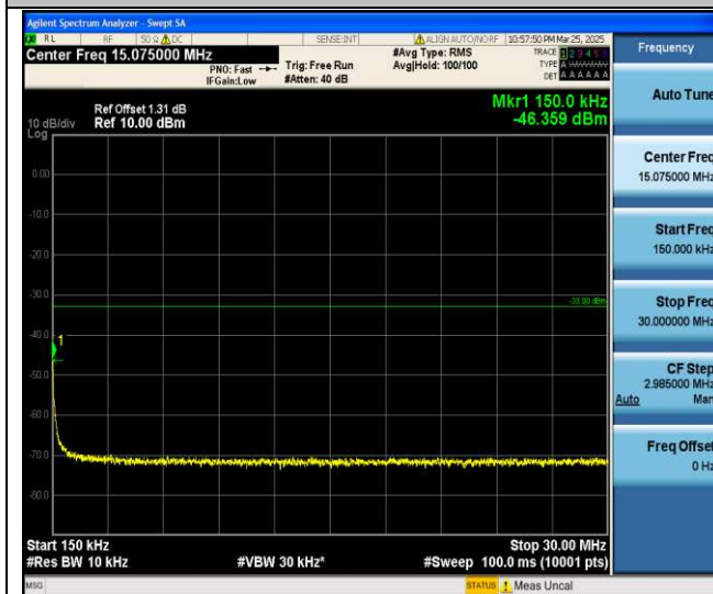
EGPRS1900-810-2-0.15~30MHz-PASS
