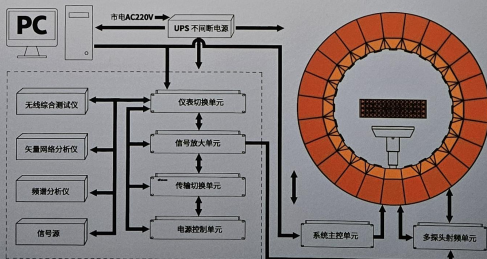
系统原理图
