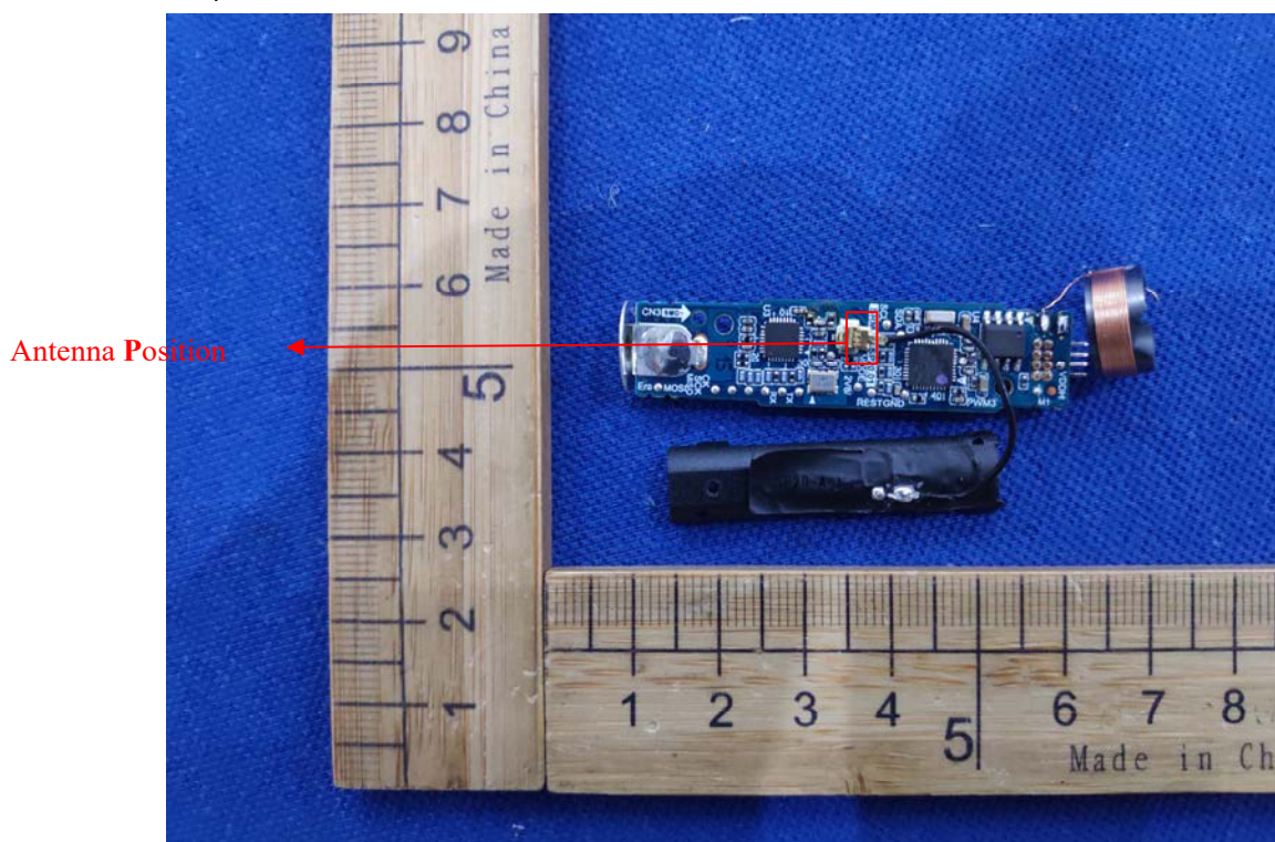
4) EUT Photo
