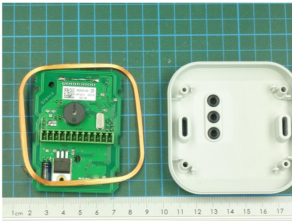
181073eut20: PRD5/2 EUT inside view 2
