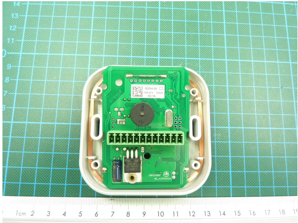
181073eut7.JPG: KPD5/2 EUT inside view 1
