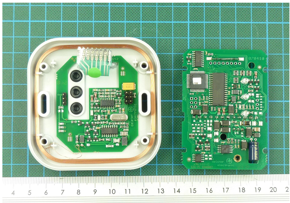
181073eut8.JPG: KPD5/2 inside view 2
