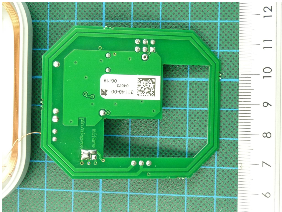
181073eut10.JPG: KPD5/2 PCB 1 bottom view
