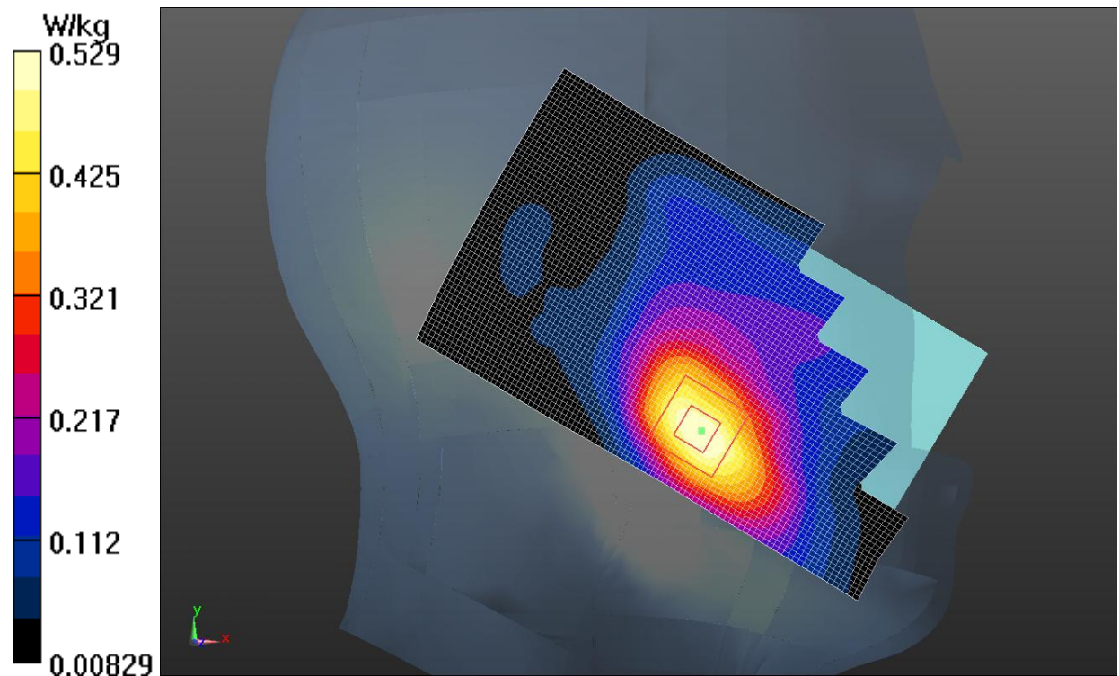
Fig.9 WCDMA1700
