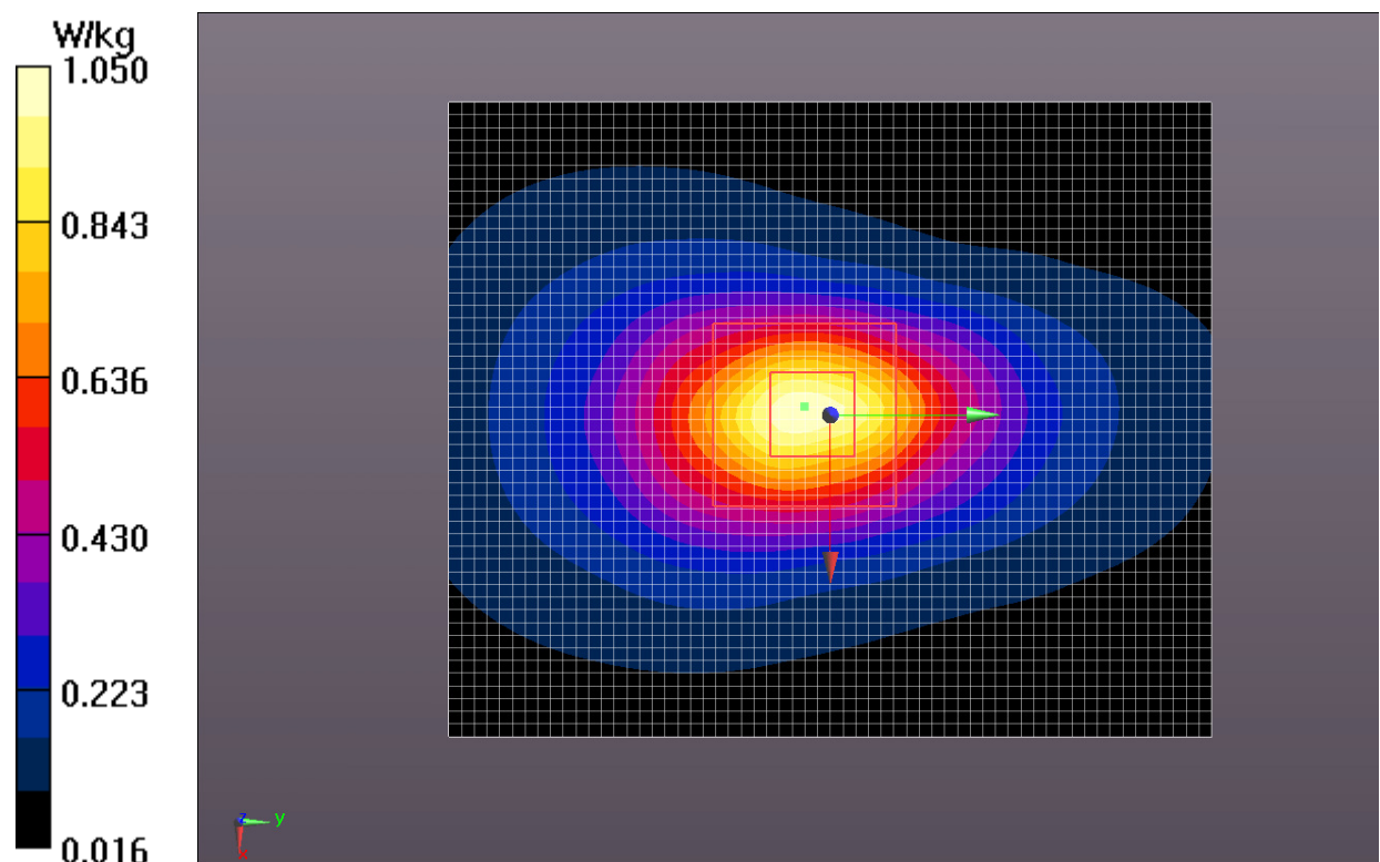
Fig.8 WCDMA1900 CH9538
