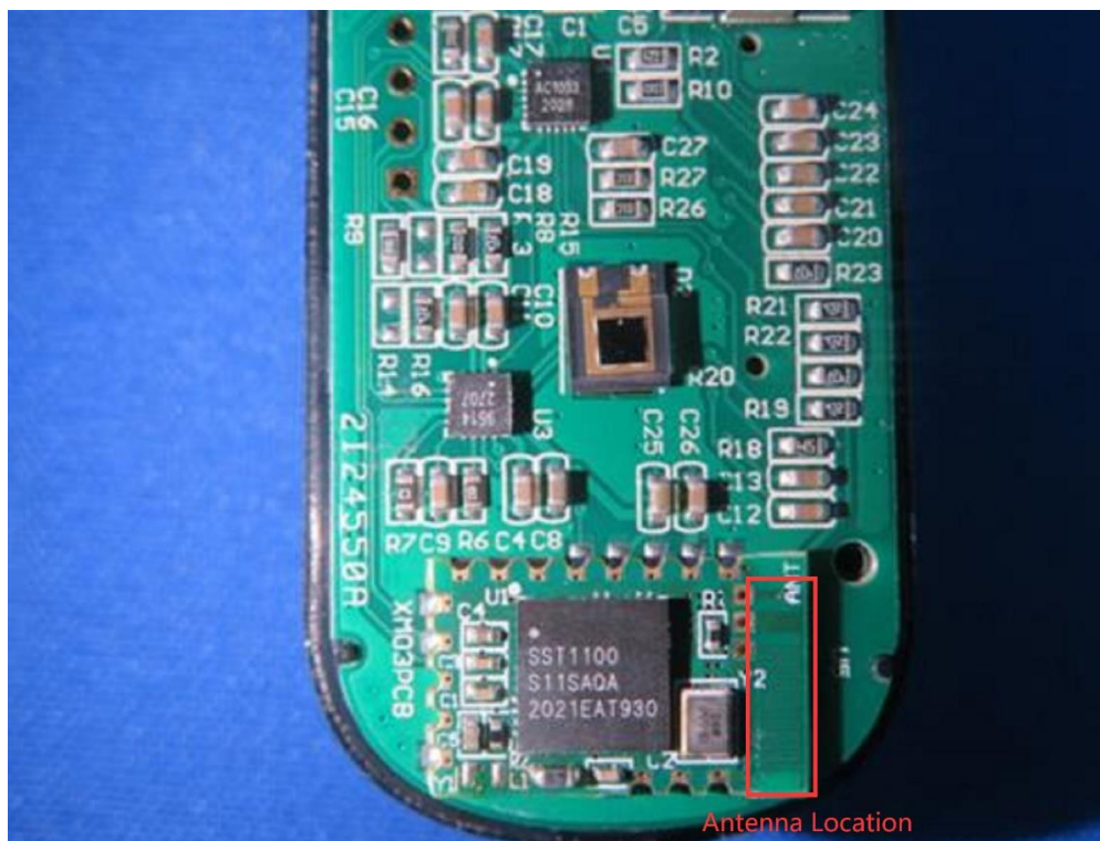
(8) EUT Photo
