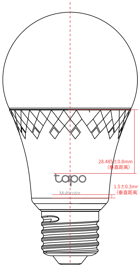
结构图
