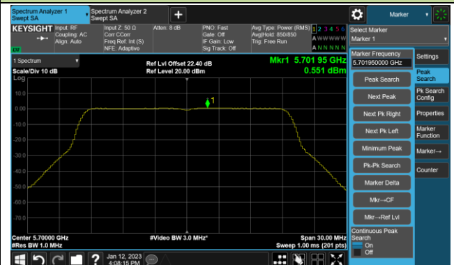
Channel 140 (5700MHz)
