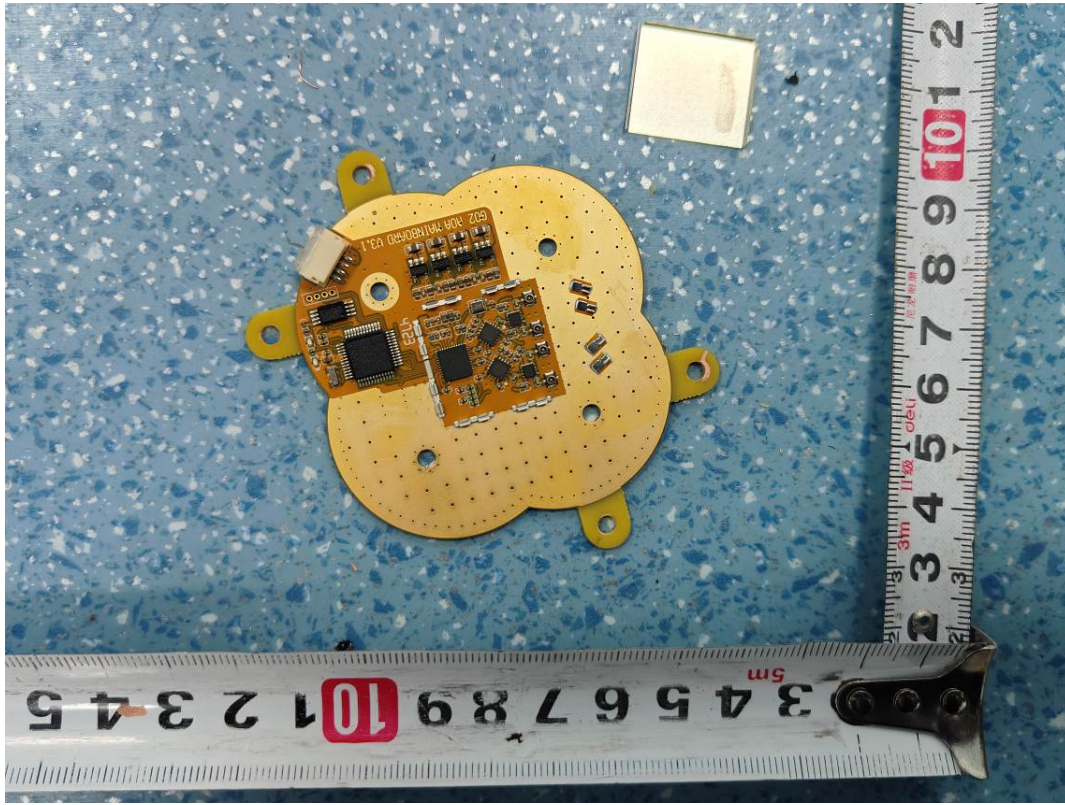
UWB Chip
