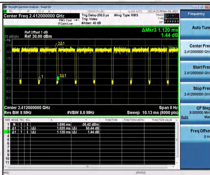
11AX20SISO_Ant2_2412
