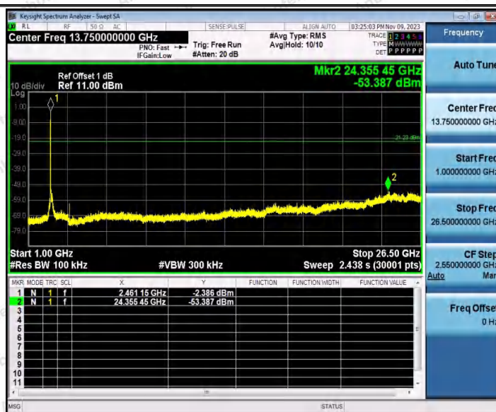
11AX20SISO_Ant2_2462_0~Reference
