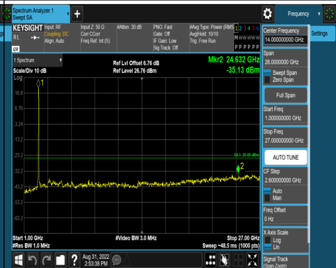
Band41-20MHz-64QAM-41490-100RB#0-Range2:100 0~27000MHz
