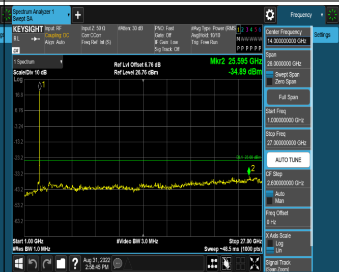
Band41-20MHz-64QAM-41490-100RB#0-Range2:100 0~27000MHz
