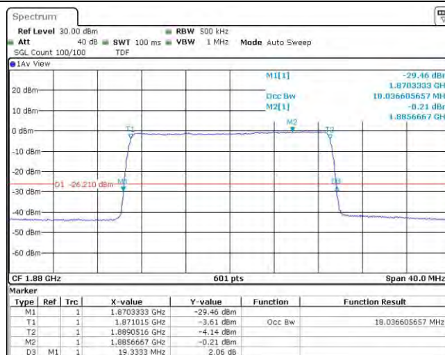
Band2-20MHz-QPSK-19100-100RB#0
