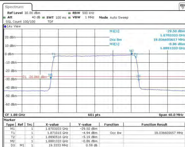
Band2-20MHz-16QAM-19100-100RB#0
