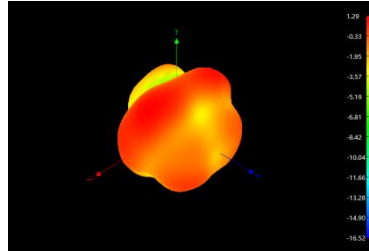
2400MHz
