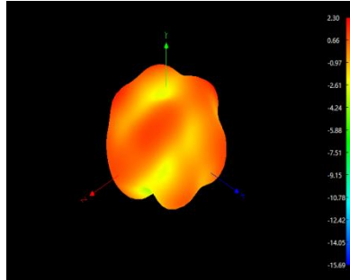
2400MHz
