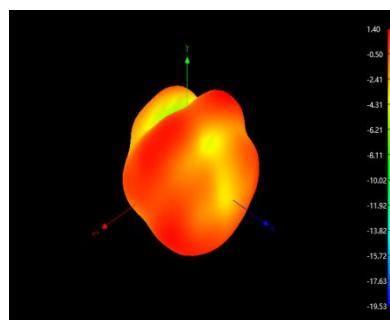
2500MHz
