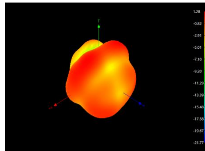
2450MHz
