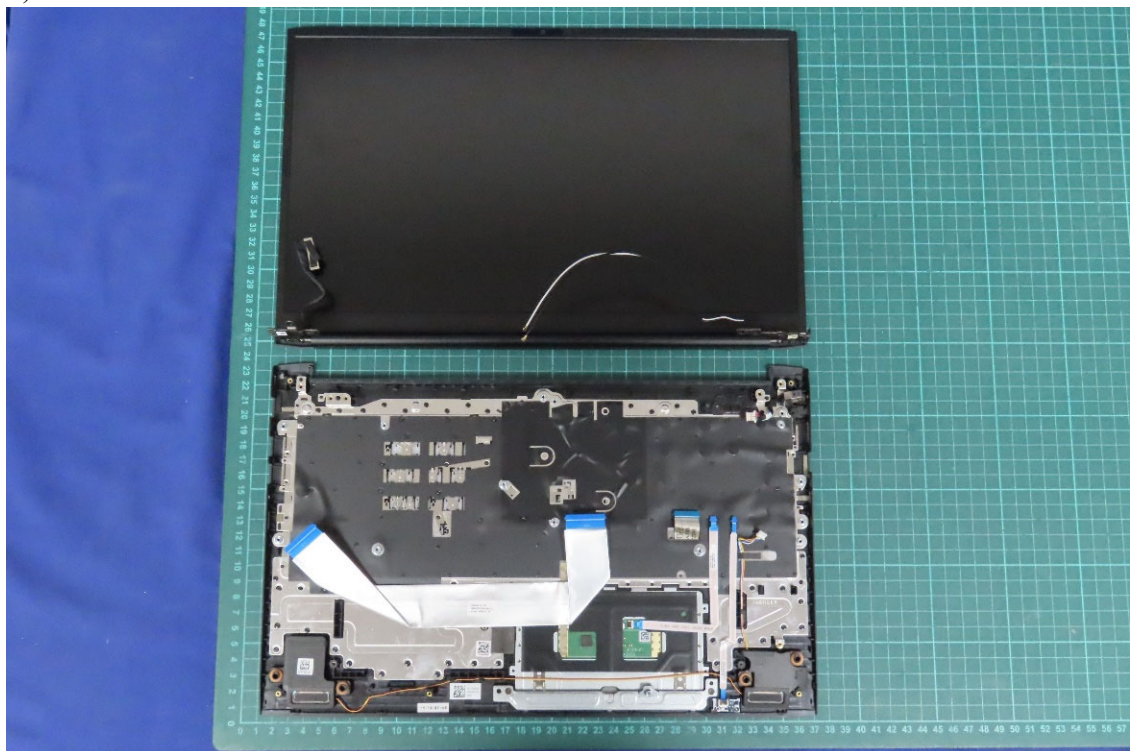
(21) EUT Photo
