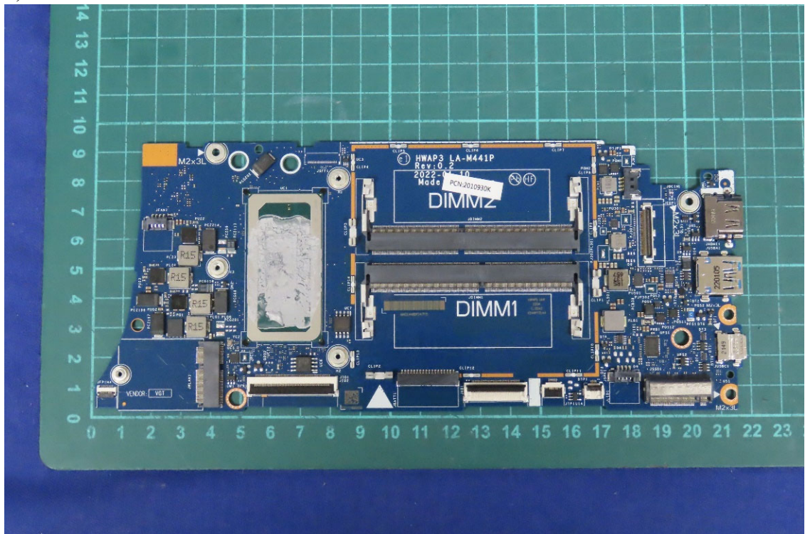
(18) EUT Photo
