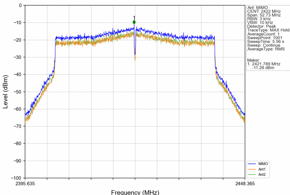
802.11be(EHT40)_LCH_2422MHz_SU_MIMO_NTNV
