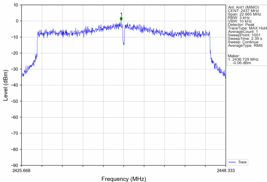
802.11be(EHT20)_MCH_2437MHz_SU_Ant1 (MIMO)_NTNV
