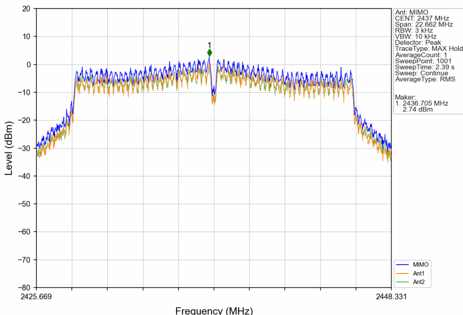
802.11n(HT20)_MCH_2437MHz_MIMO_NTNV
