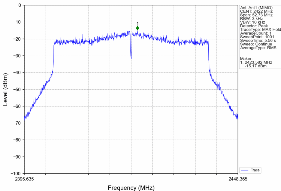
802.11be(EHT40)_LCH_2422MHz_SU_Ant1 (MIMO)_NTNV
