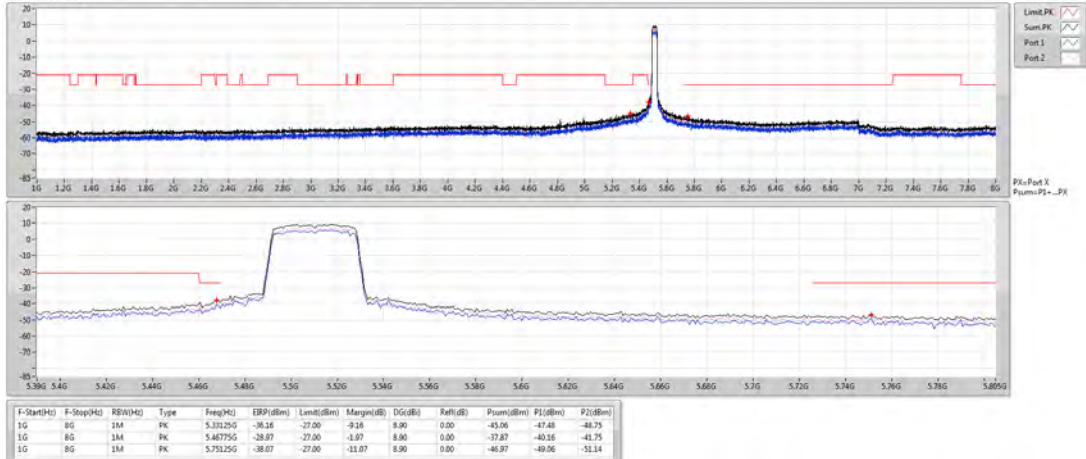
802.11ac VHT40_Nss1,(MCS0)_2TX 5510MHz
