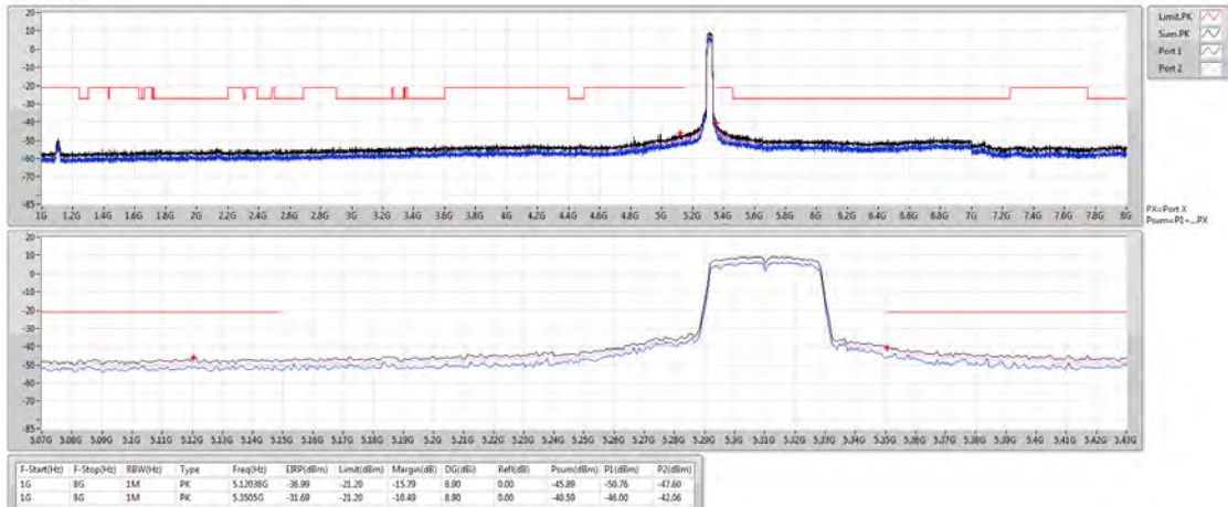
802.11ac VHT40_Nss1,(MCS0)_2TX 5310MHz
