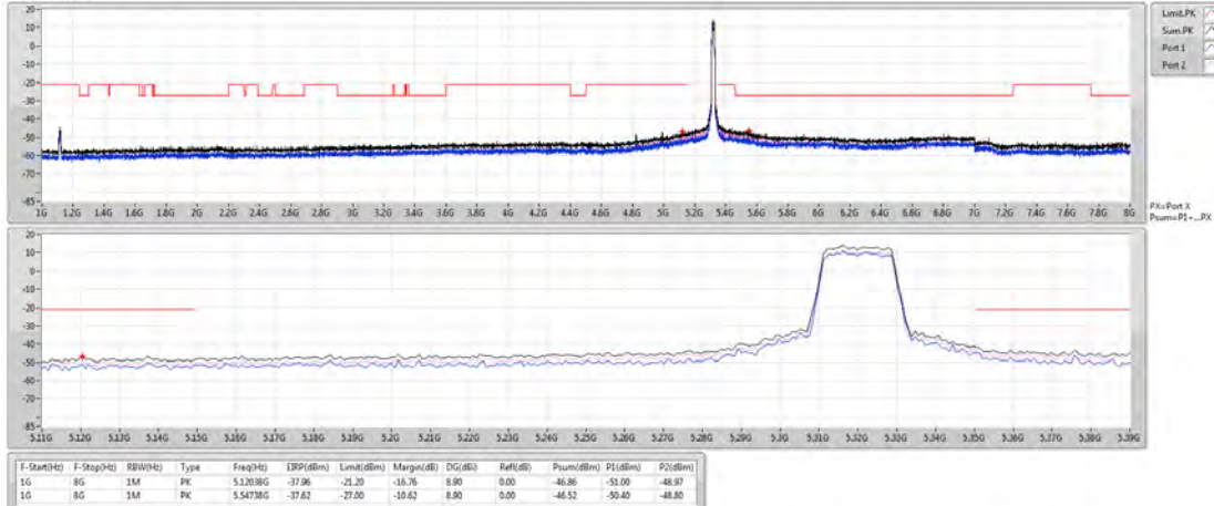
802.11ac VHT20_Nss1,(MCS0)_2TX 5320MHz
