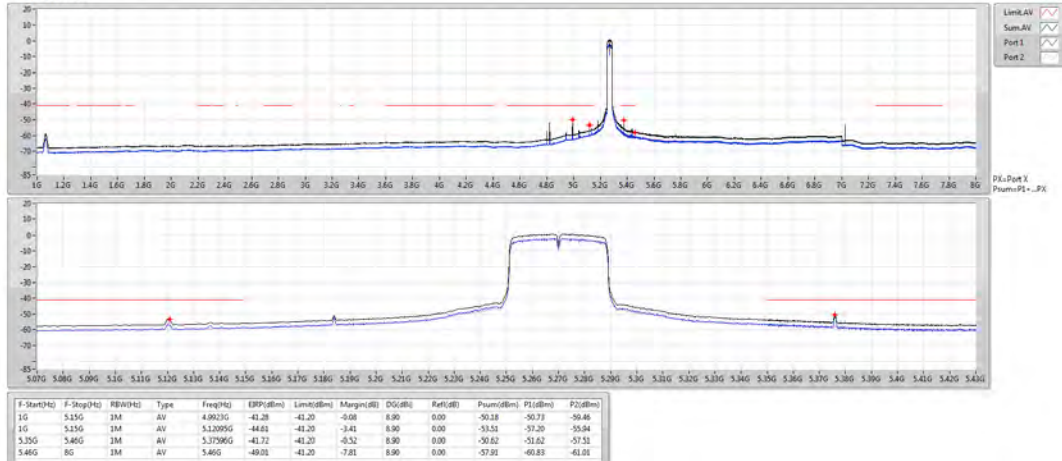
802.11ac VHT40_Nss1,(MCS0)_2TX 5270MHz
