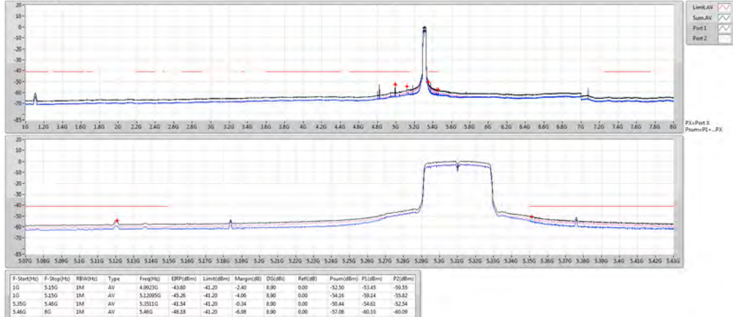
802.11ac VHT40_Nss1,(MCS0)_2TX 5310MHz
