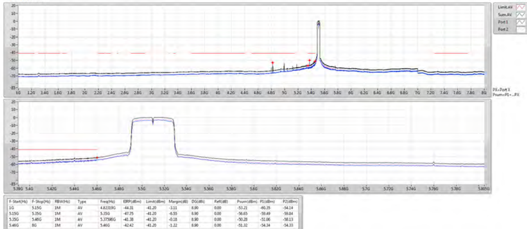
802.11ac VHT40_Nss1,(MCS0)_2TX 5510MHz
