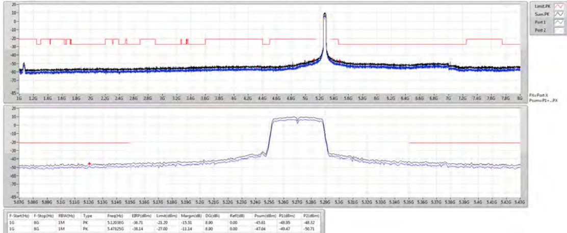
802.11ac VHT40_Nss1,(MCS0)_2TX 5270MHz
