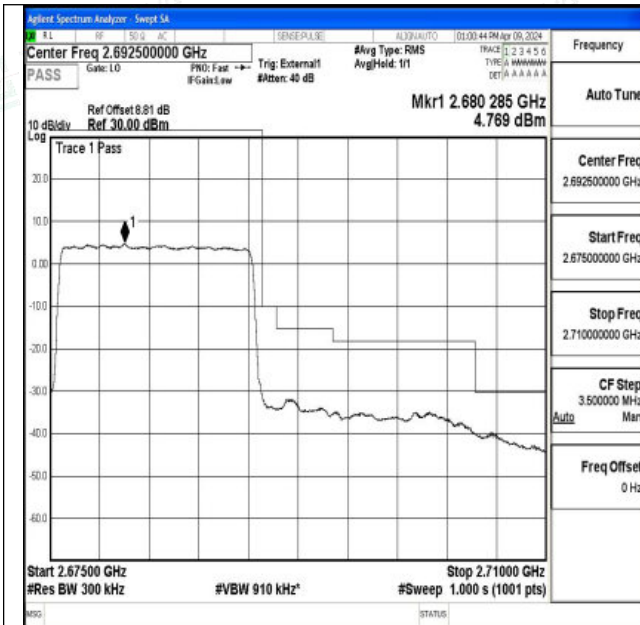
Band41_15MHz_QPSK_41515_75RB#0
