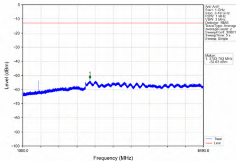
n5 30kHz SISO NTN 15MHz CP-OFDM QPSK 836.5MHz Edge 1RB Left
