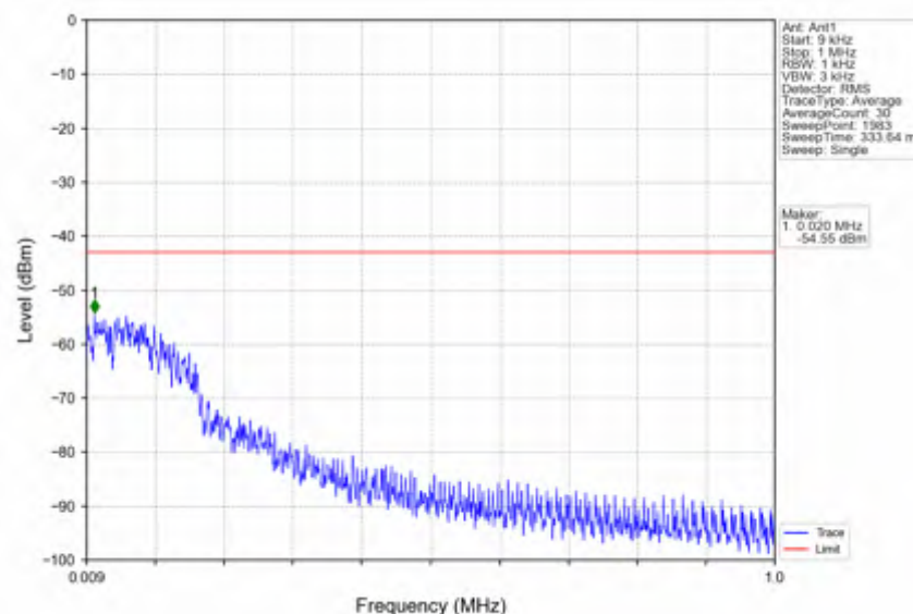
n5 15kHz SISO NTV 20MHz CP-OFDM QPSK 836.5MHz Edge 1RB Left
