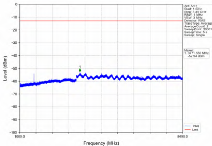
n5 30kHz SISO NTNv 20MHz DFT-s-OFDM QPSK 834MHz Edge 1RB Left
