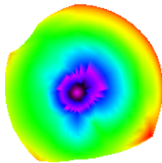
5150.000MHz
