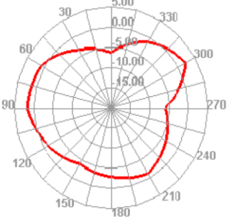
5500.000MHz E2
