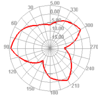
5500.000MHz E1
