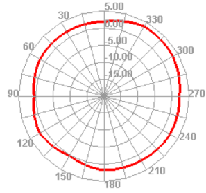
2450.000MHz H
