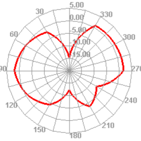
2450.000MHz E1
