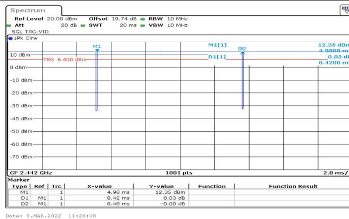
11G_Ant1_2442
