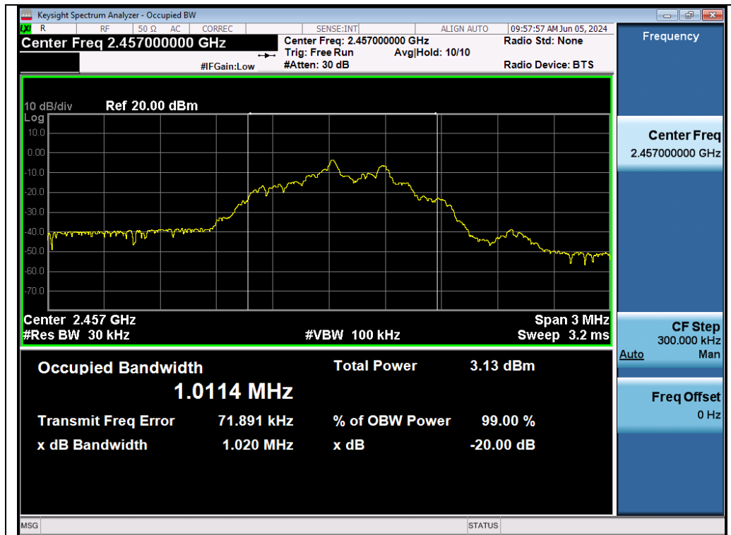
Test_Graph_GFSK_ANT1_2457_OBW
